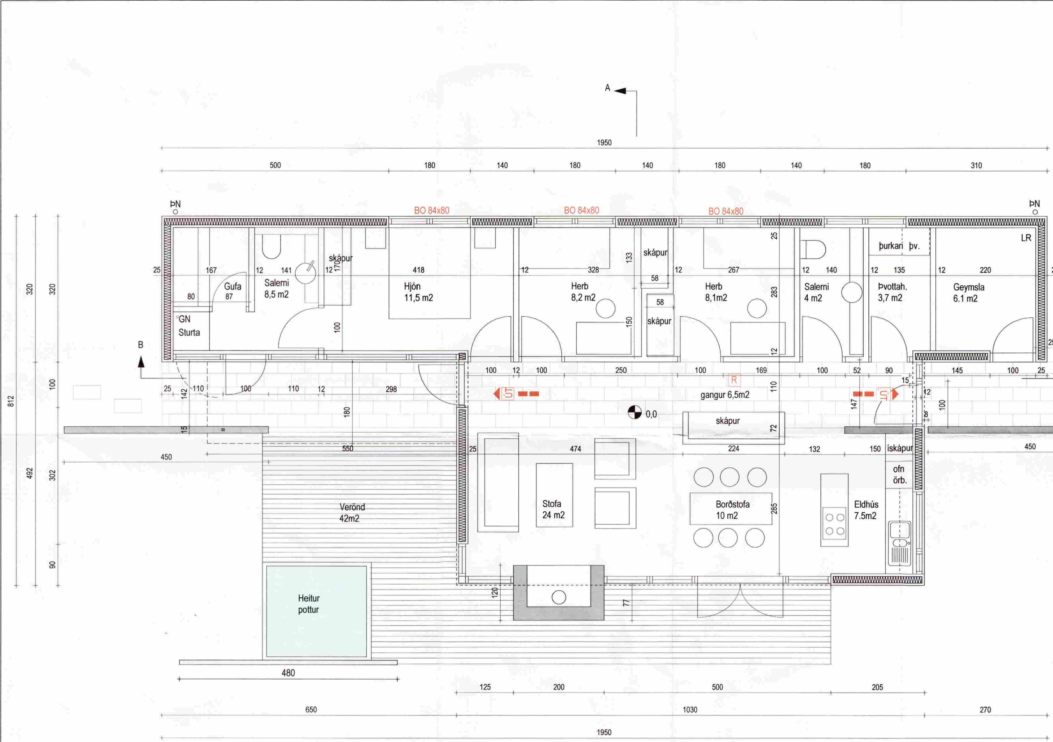
Grunnmynd 1:50
