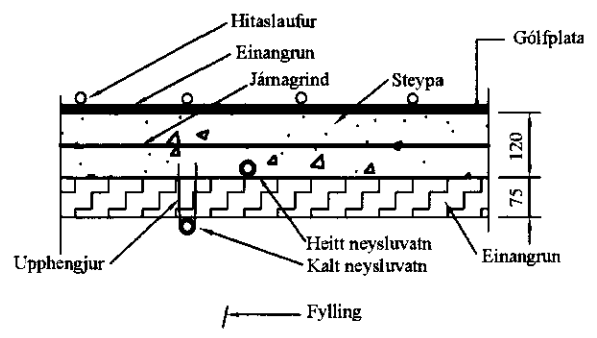
EINKENNANDI SNIÐ Í GÓLFPLÖTU 1:10
