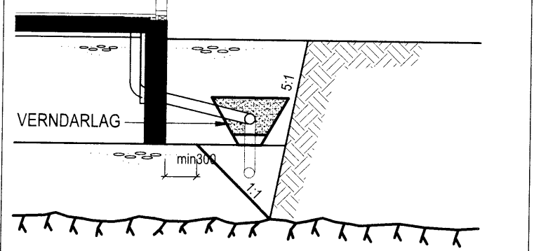
SNID VIÐ SÖKKUL Mkv. 1:50
