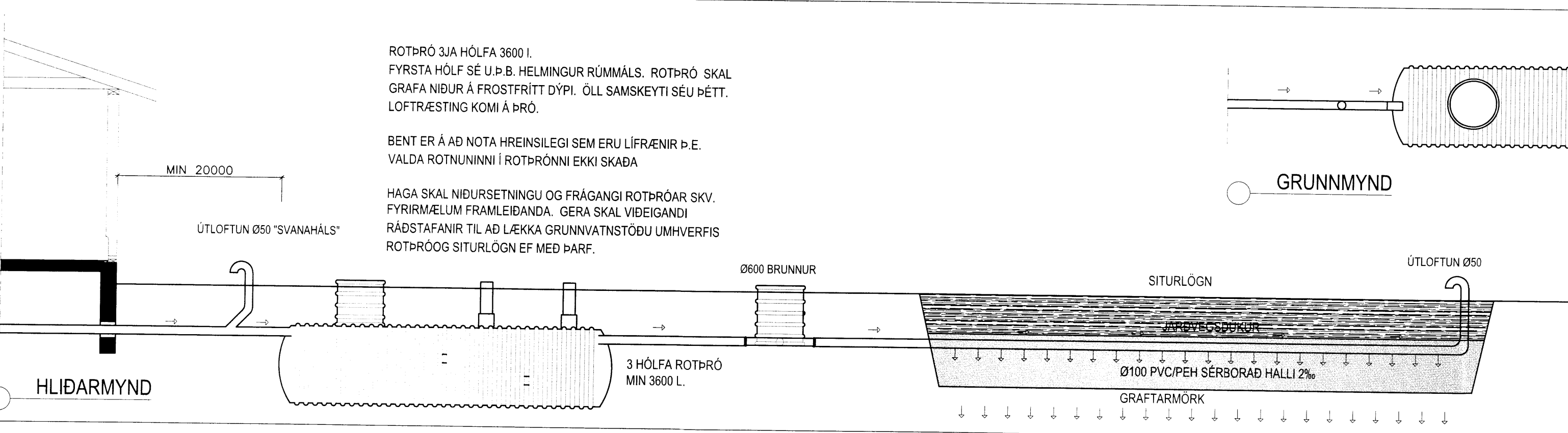
GRUNNMYND FRÆNNISLAGNA Mkv. 1:50
