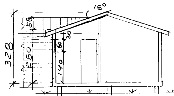
SNITT A-A
