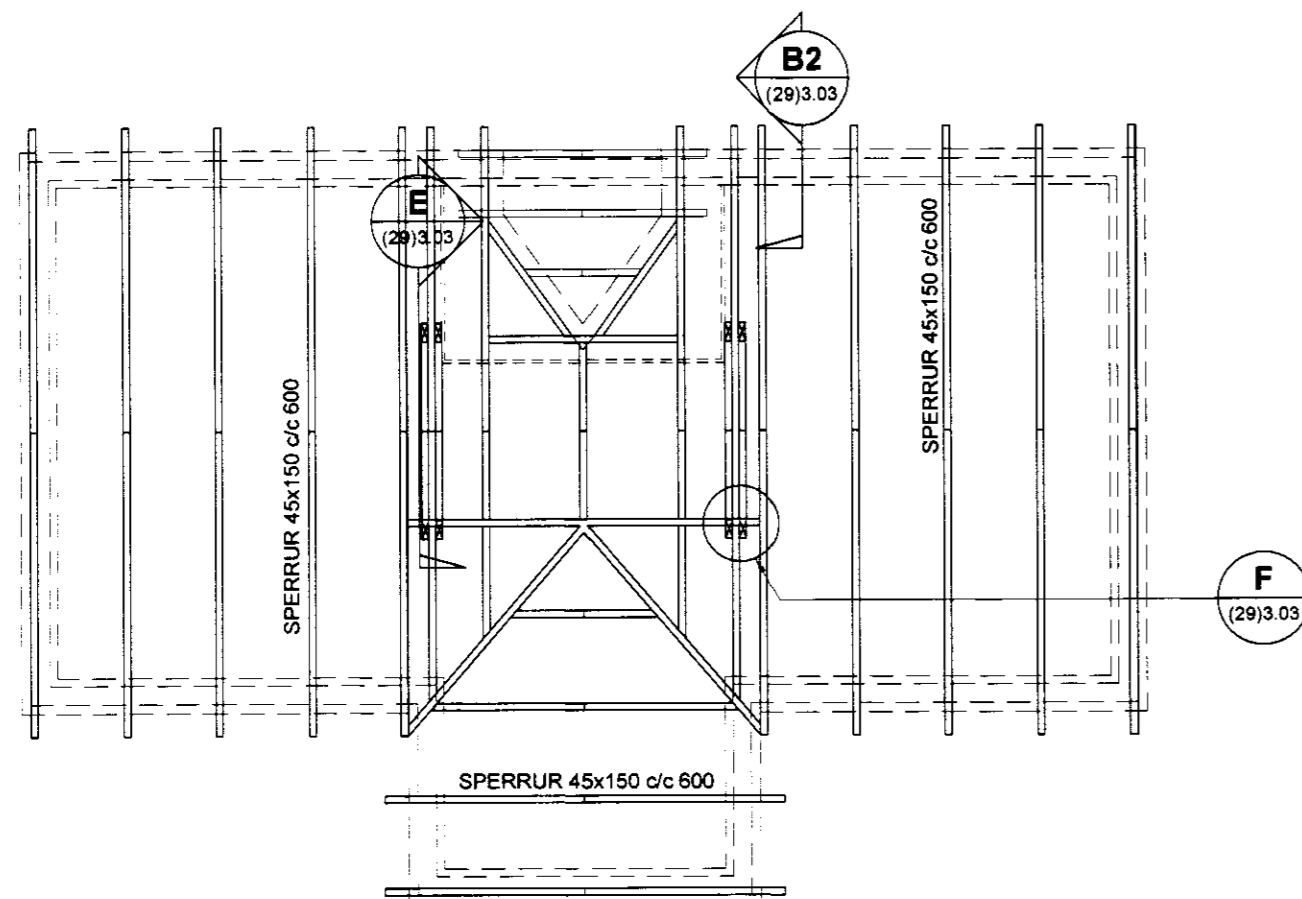
SPERRUPLAN Í MKV.: 1: 50
