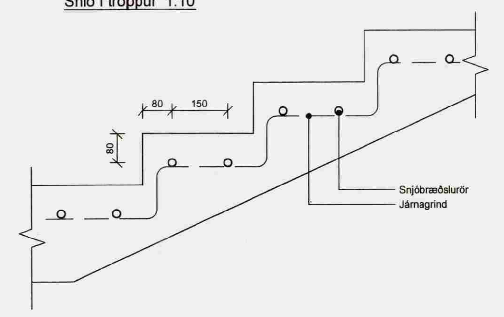
Snið í tröppur 1:10
