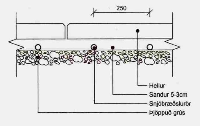
Snið í hellur 1:10
