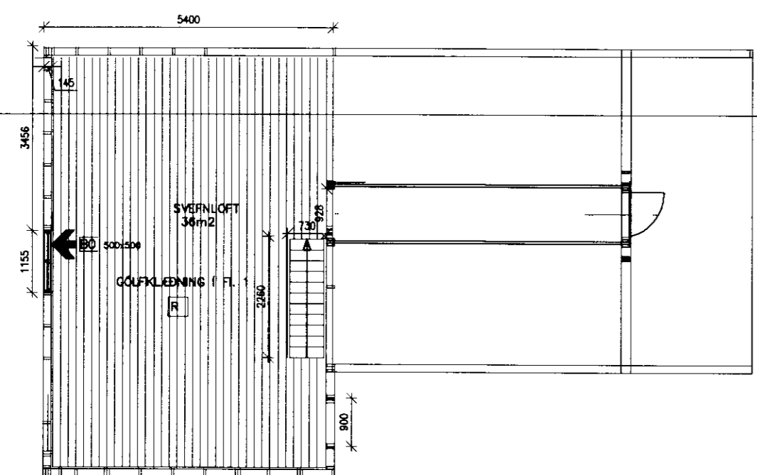
GRUNNMYND SVEFNLOFTS M.1:100
