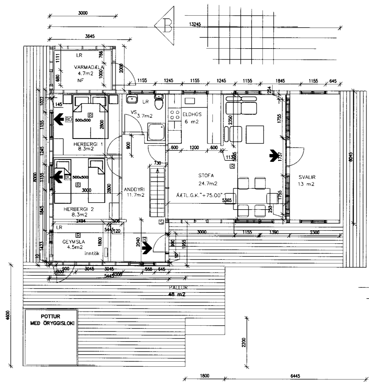
GRUNNMYND AÐALHÆÐ M.1:100
