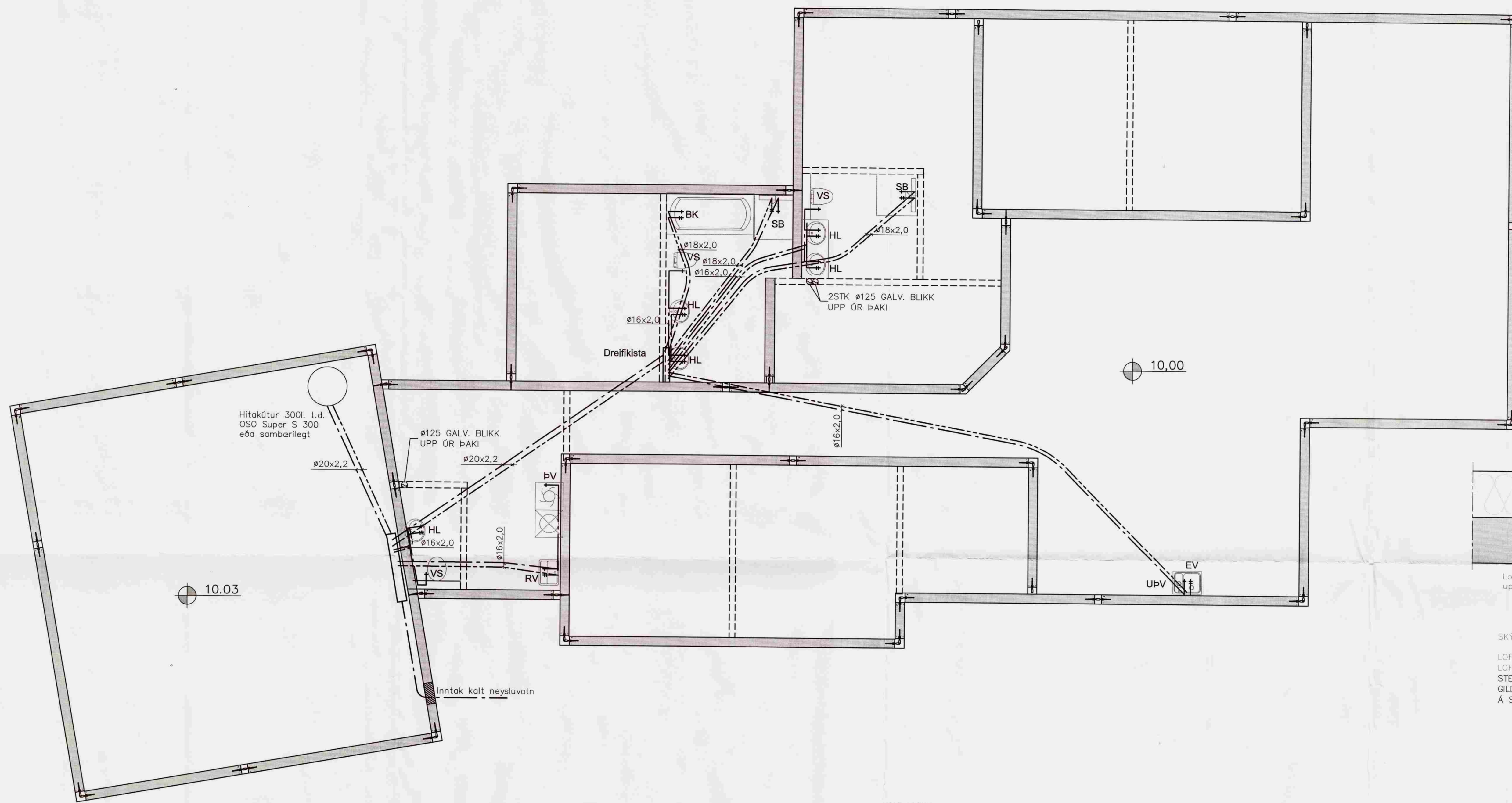
Grunnmynd neysluvatnslagna 1:50
