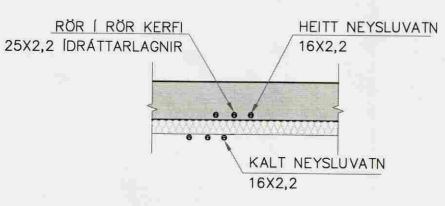
Snið í botnplötu 1:20
