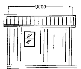
GAFL GUFUBAD KVARÐI 1:100 VESTURHLIÐ
