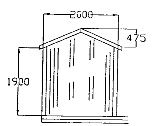
GAFL GUFUBAD KVARÐI 1:100 VESTURHLIÐ
