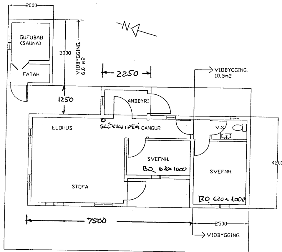
GRUNNMYND KVARÐI 1:100
