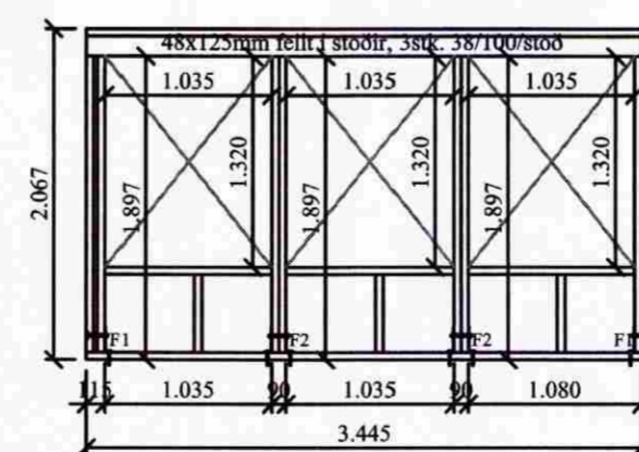
Grind nr. 3 - 48x125mm Ath: Öll mál þarf að sannreyna á staðnum - skoða þarf sérstaklega glugga og hurðamál
