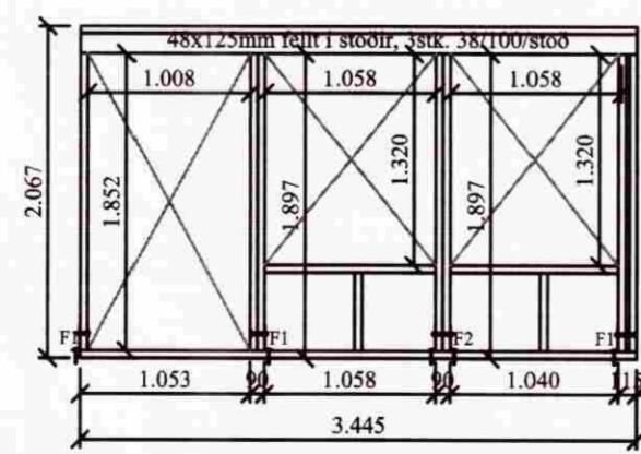
Grind nr. 1 - 48x125mm Ath: Öll mál þarf að sannreyna á staðnum - skoða þarf sérstaklega glugga og hurðamál
