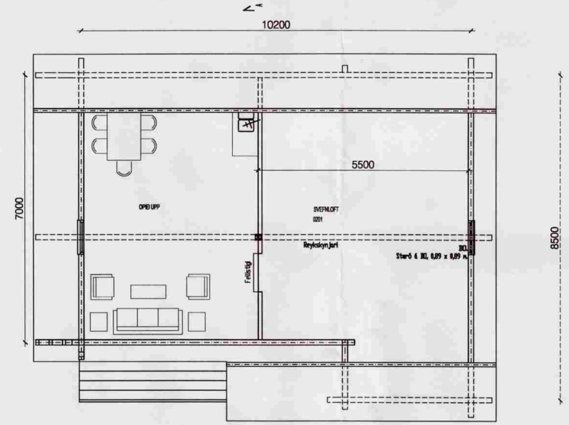
GRUNNMYND, SVEFNLOFT
