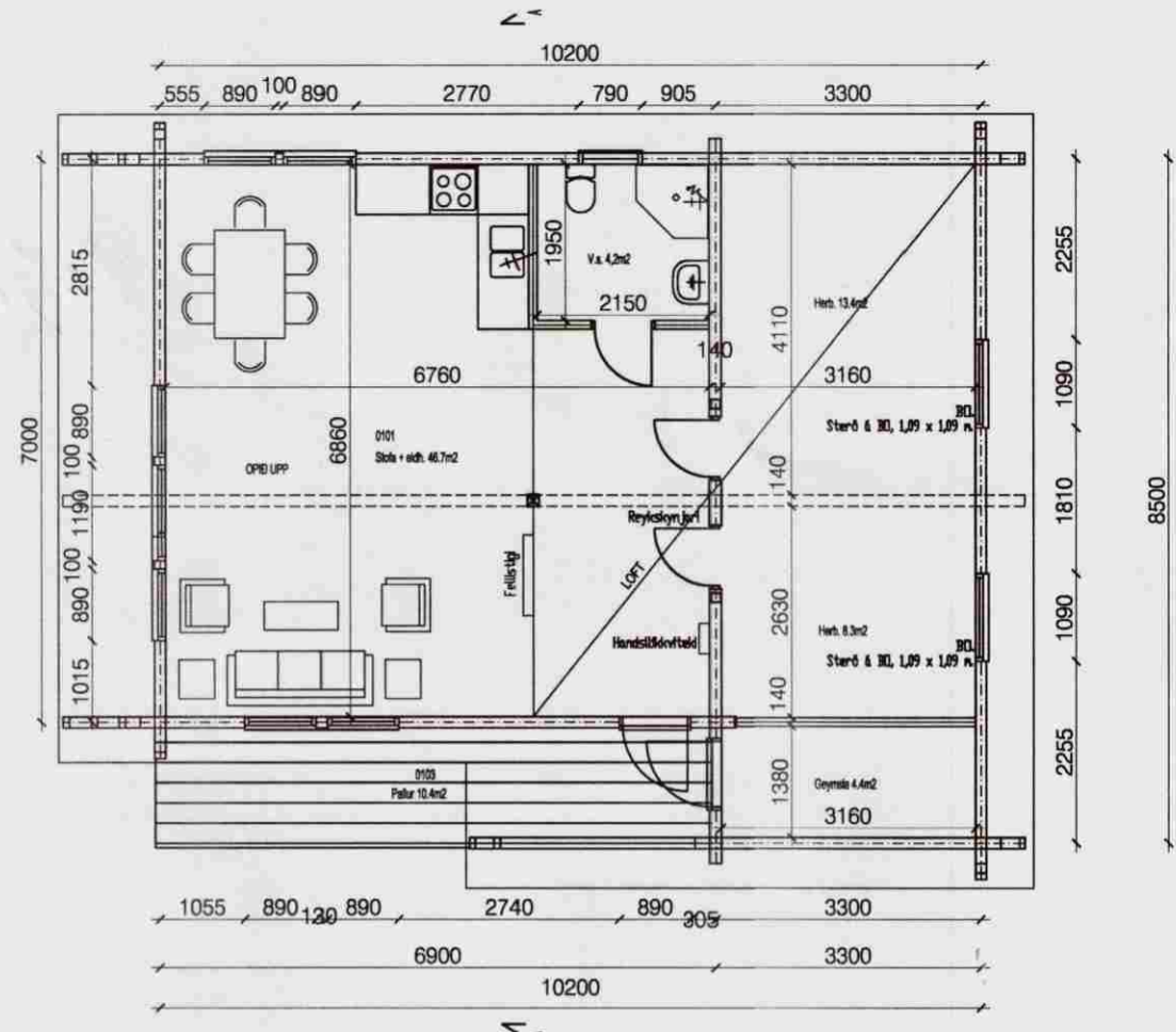
GRUNNMYND
