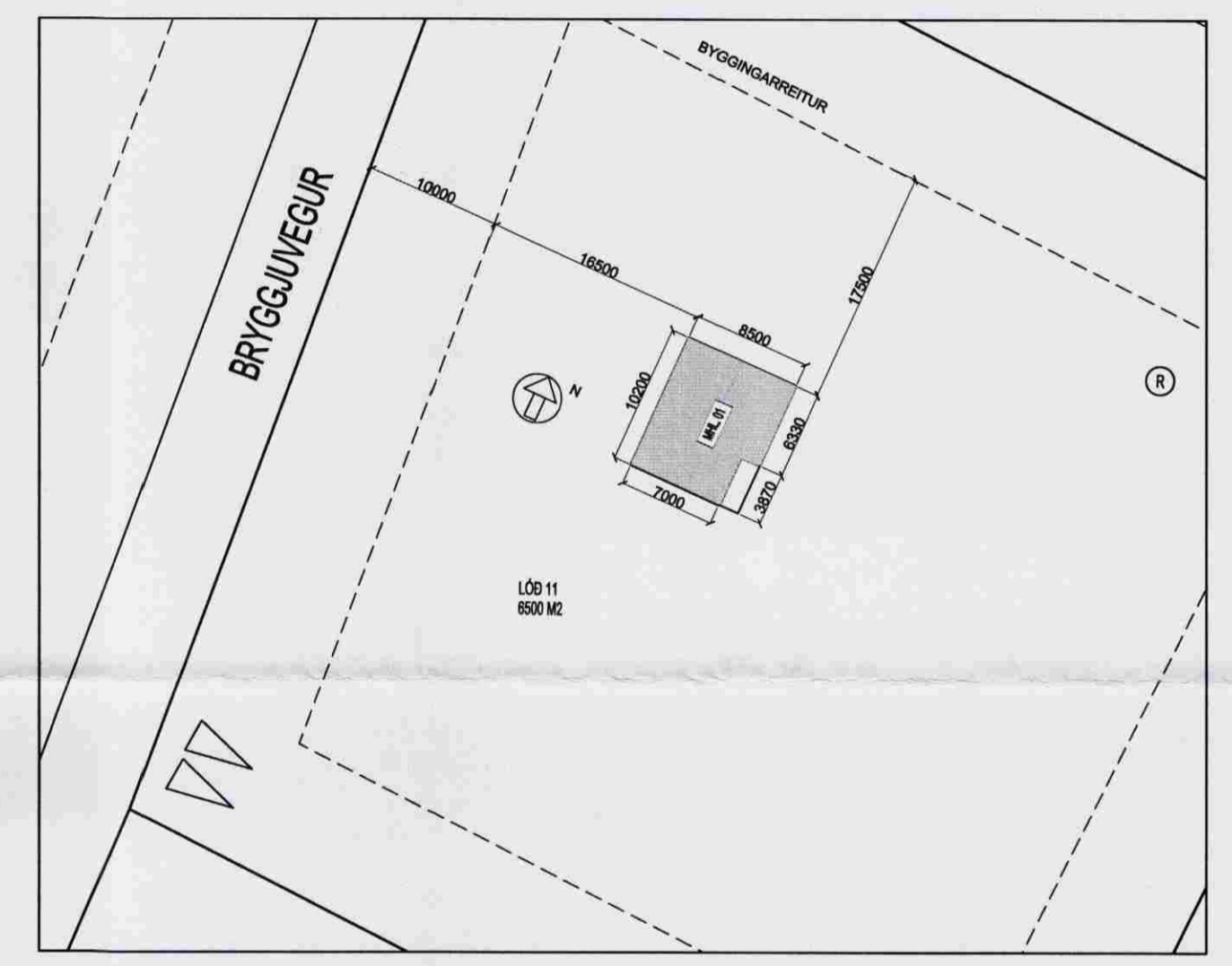
AFSTAÐA 1:500
