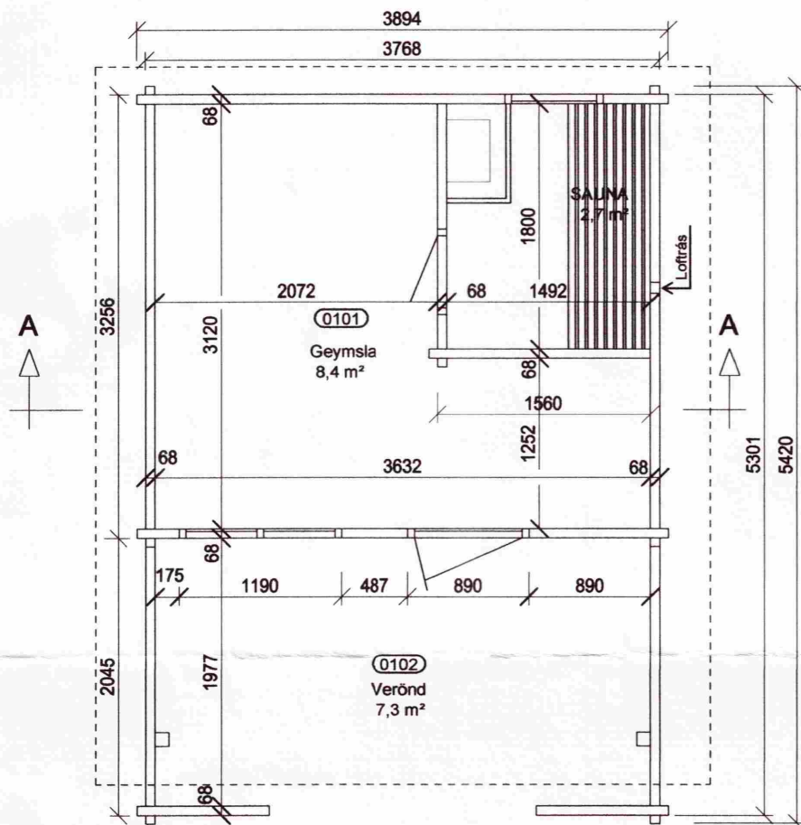
GRUNNMYND
