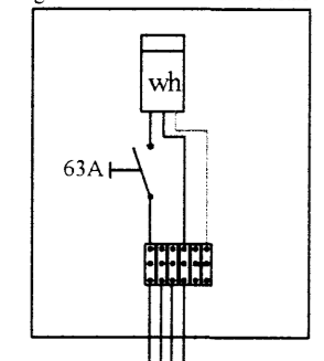
Innsiglaður mælakassi utan á bústað
