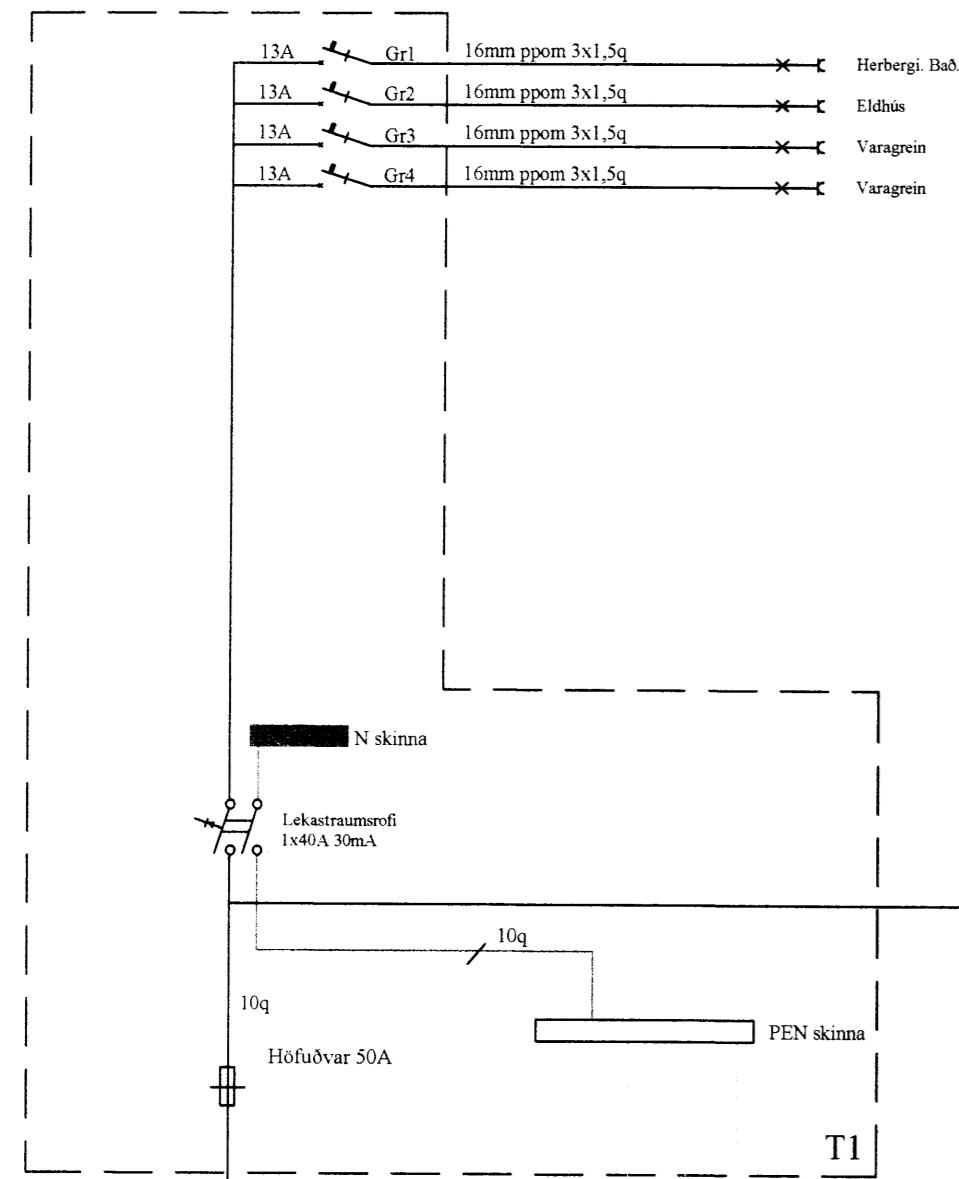
Innsiglaður mælakassi utan á bústað
