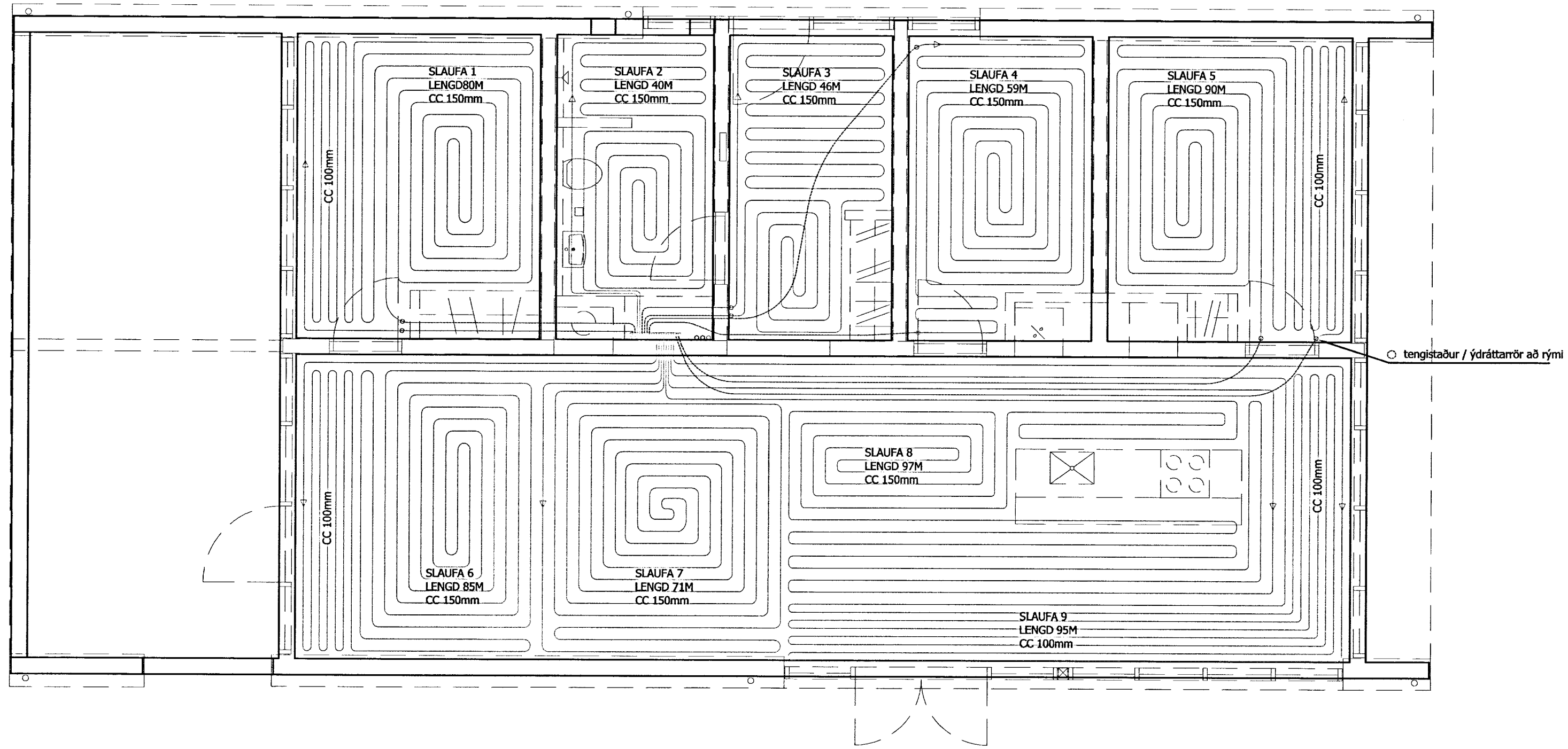
GRUNNMYND GÓLFGEYSLA 1:50
