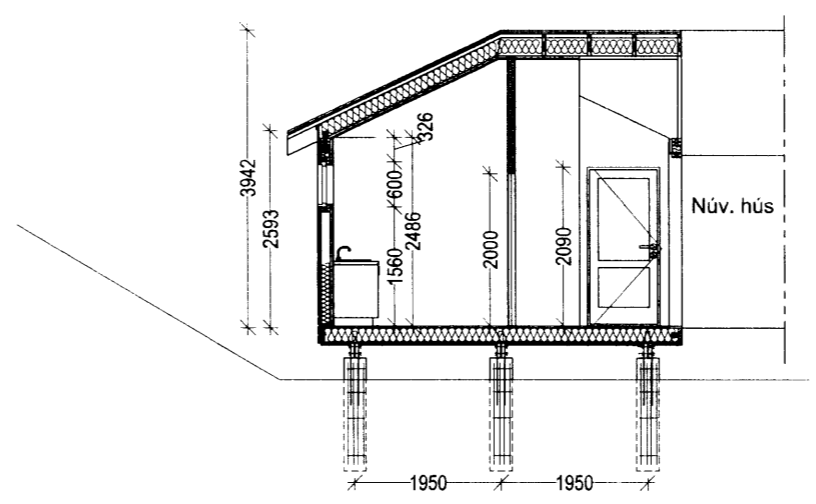
Snið B-B
