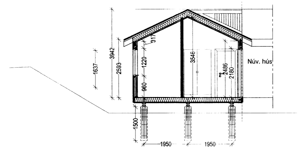
Snið A-A
