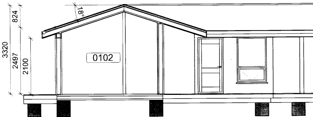
A Snið M 1:100
