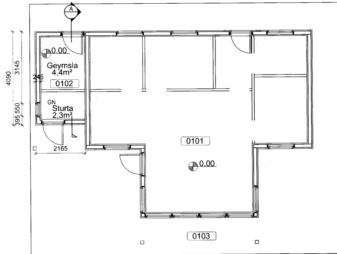
GRUNNMYND mkv. 1:100
