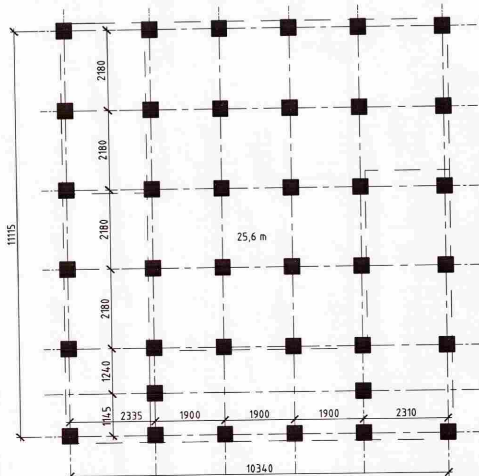
UNDIRSTÖÐUR 1 : 100
