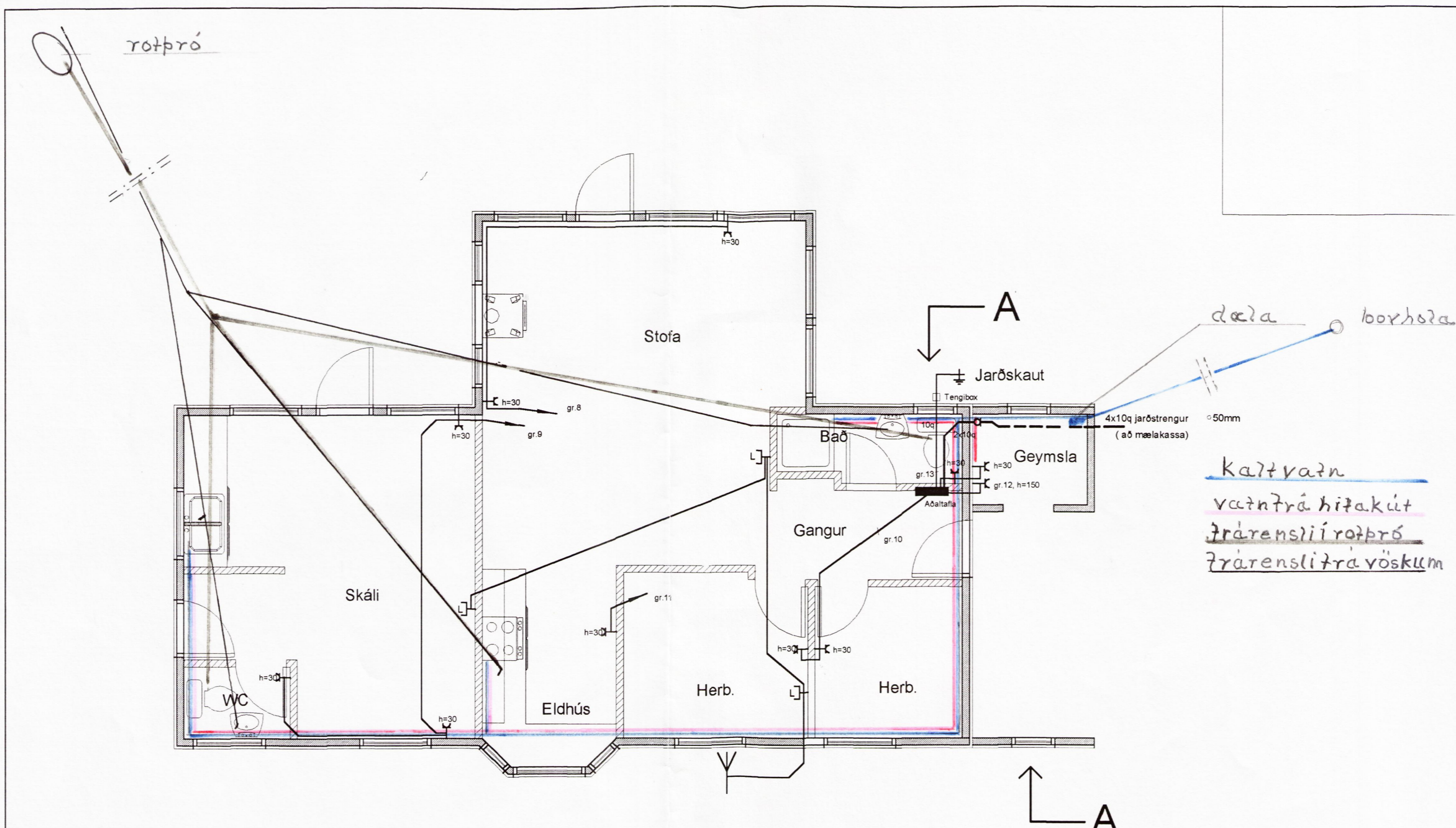
Grunnmynd 2 Mælikvarði 1:50
