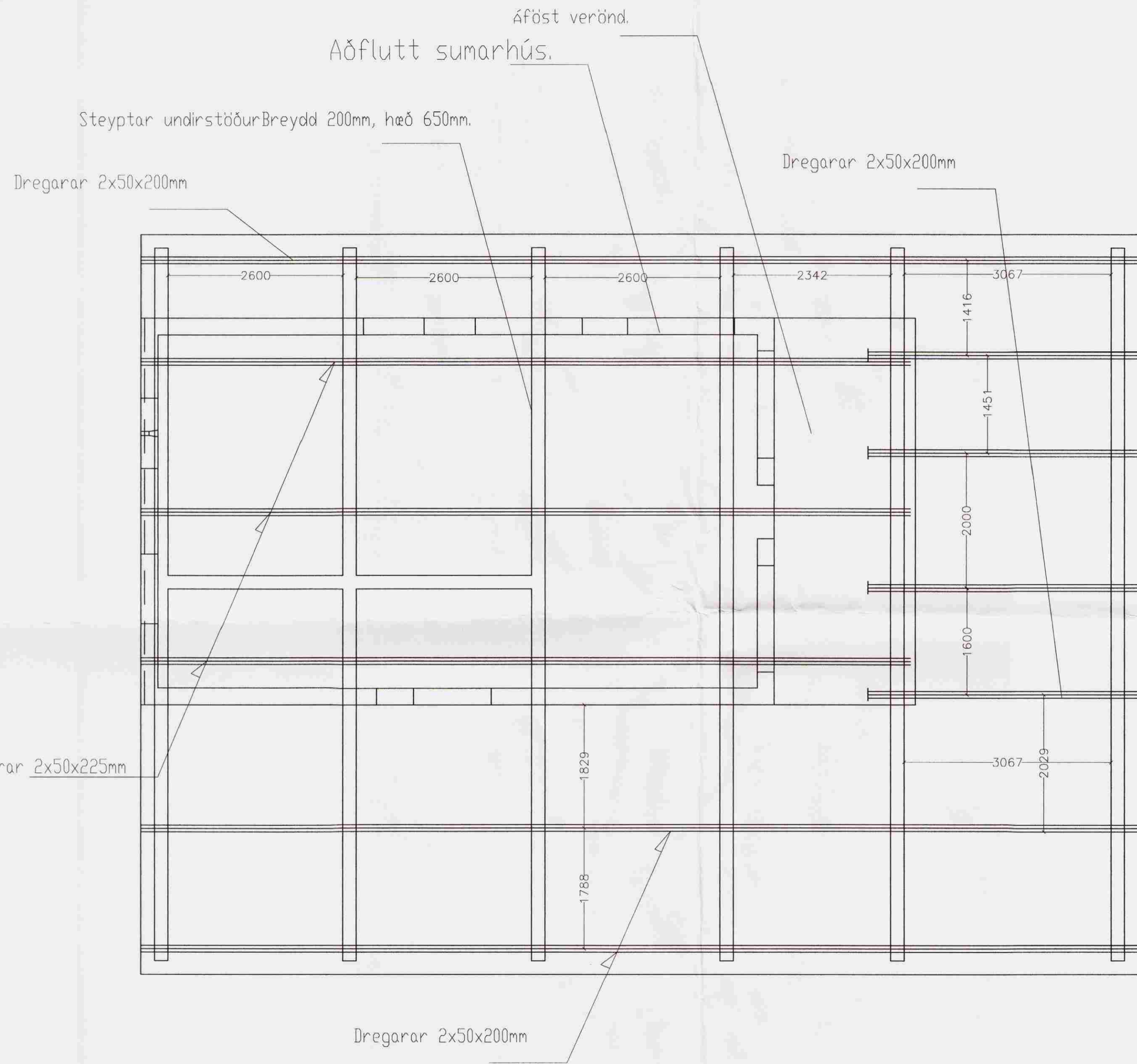
Grunnmynd 1:50
