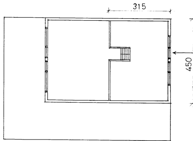
GRUNNMYND SVEFNLOFTS MKV. 1:100
