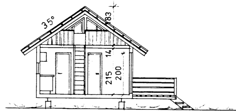
SNIÐ MKV. 1:100
