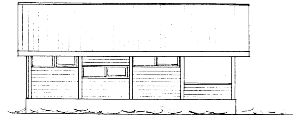
HLIÐ D
