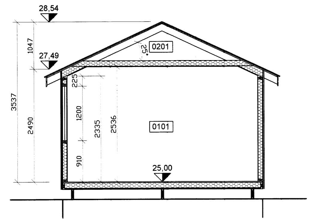
○ Snið A - 1:50
