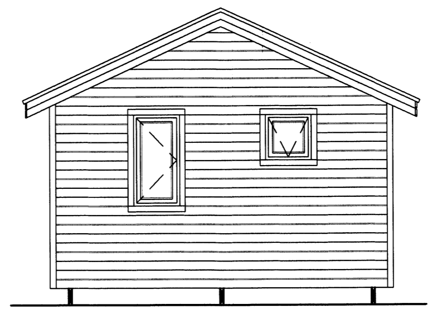
○ Norður hlið - 1:50
