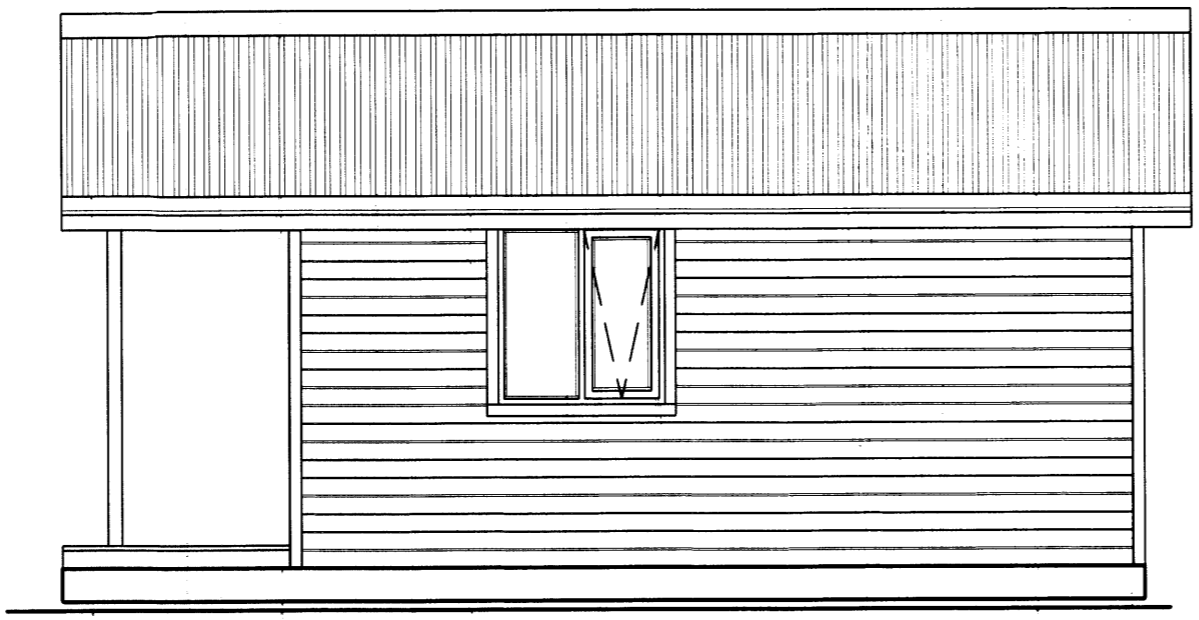
○ Austur hlið - 1:50
