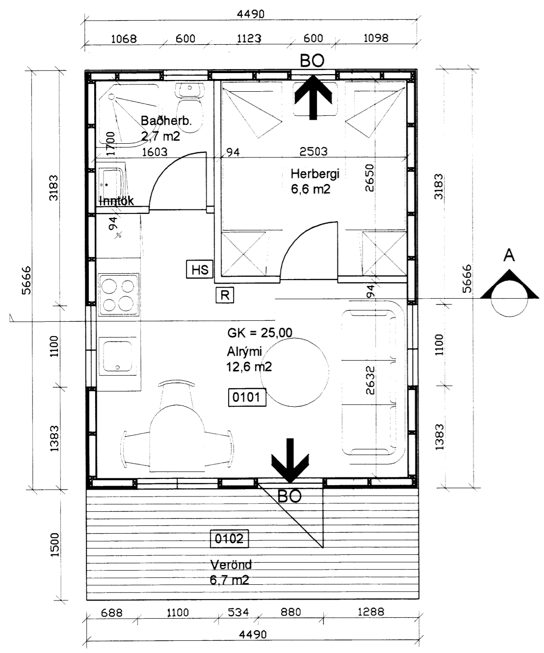
○ Grunnmynd - 1:50
