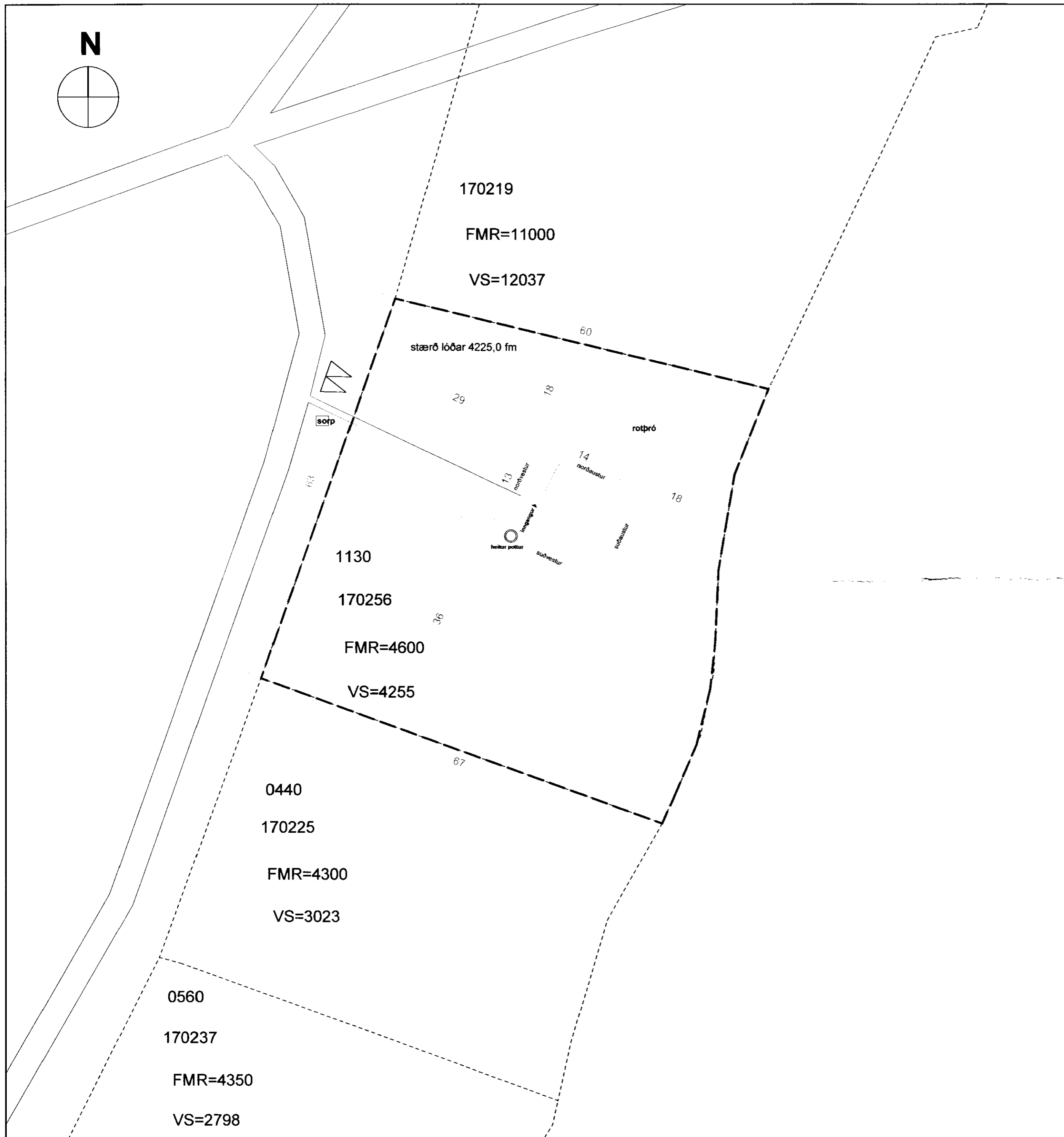
afstöðumynd 1:500
