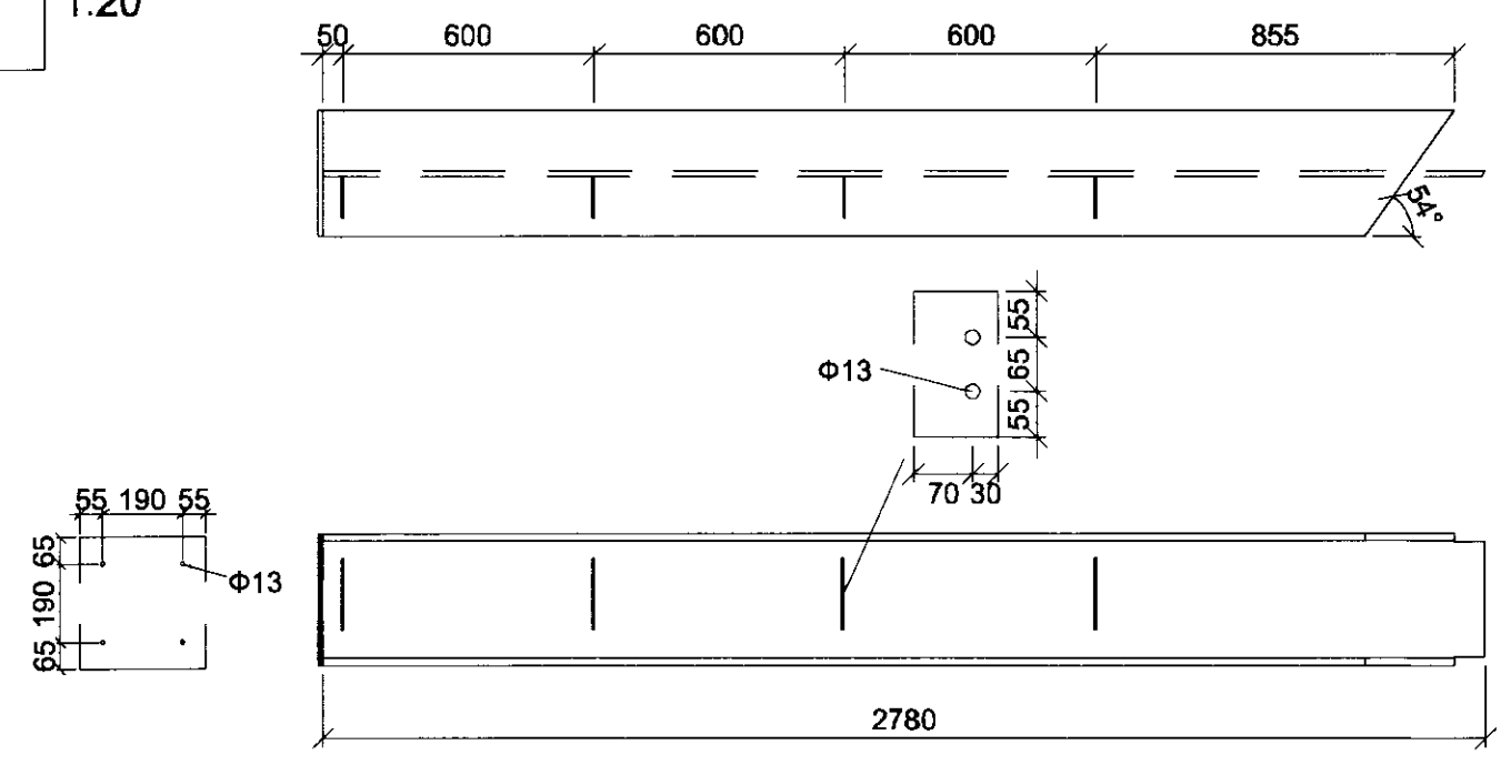
B2 Biti 201 1:20
