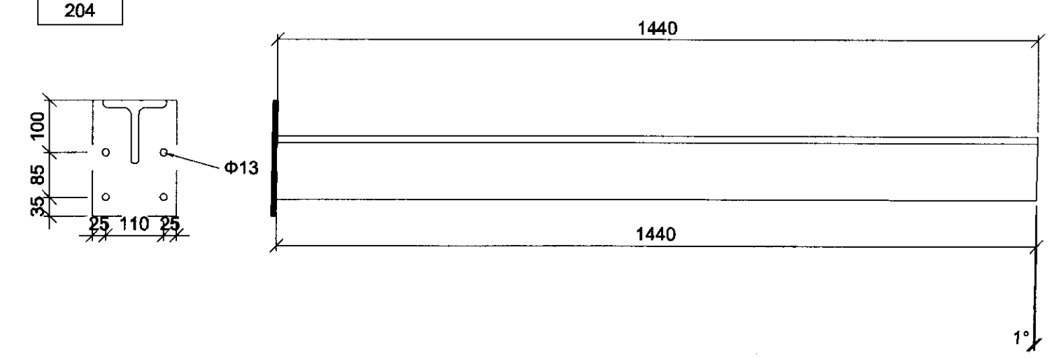
T1 Biti 201 1:10 204
