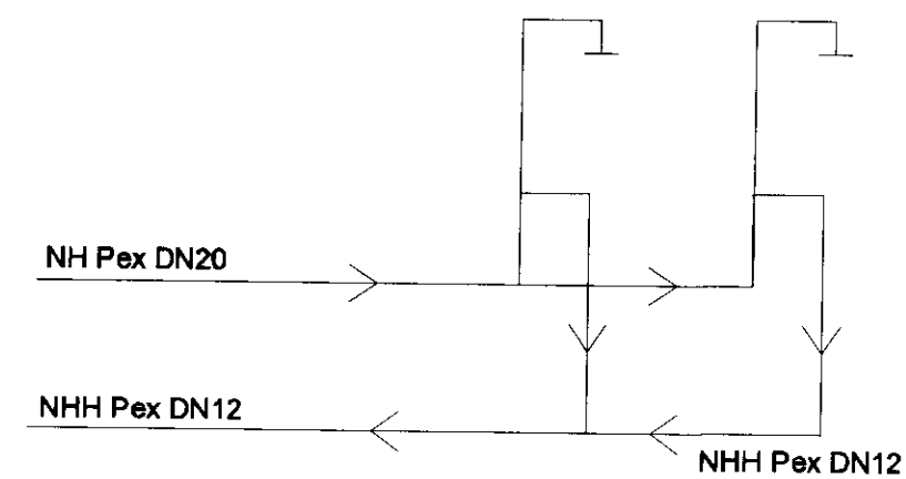
Skematisk mynd af útisturtum við gufubað
