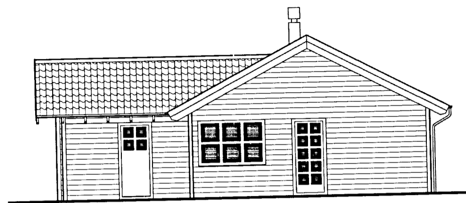
ÚTLIT SUDUR 1:100
