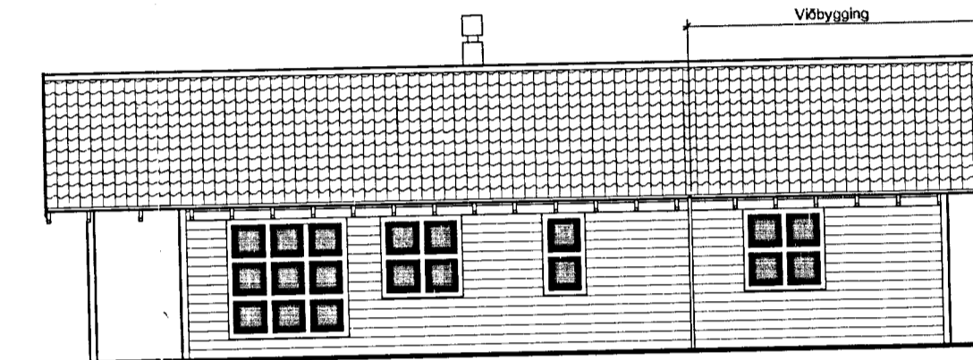
ÚTLIT AUSTUR 1:100
