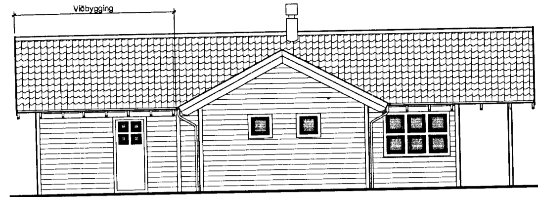
ÚTLIT VESTUR 1:100
