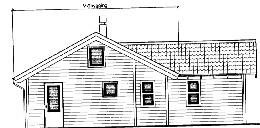
ÚTLIT NORDUR 1:100
