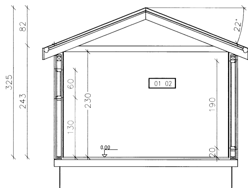
SNID A-A
