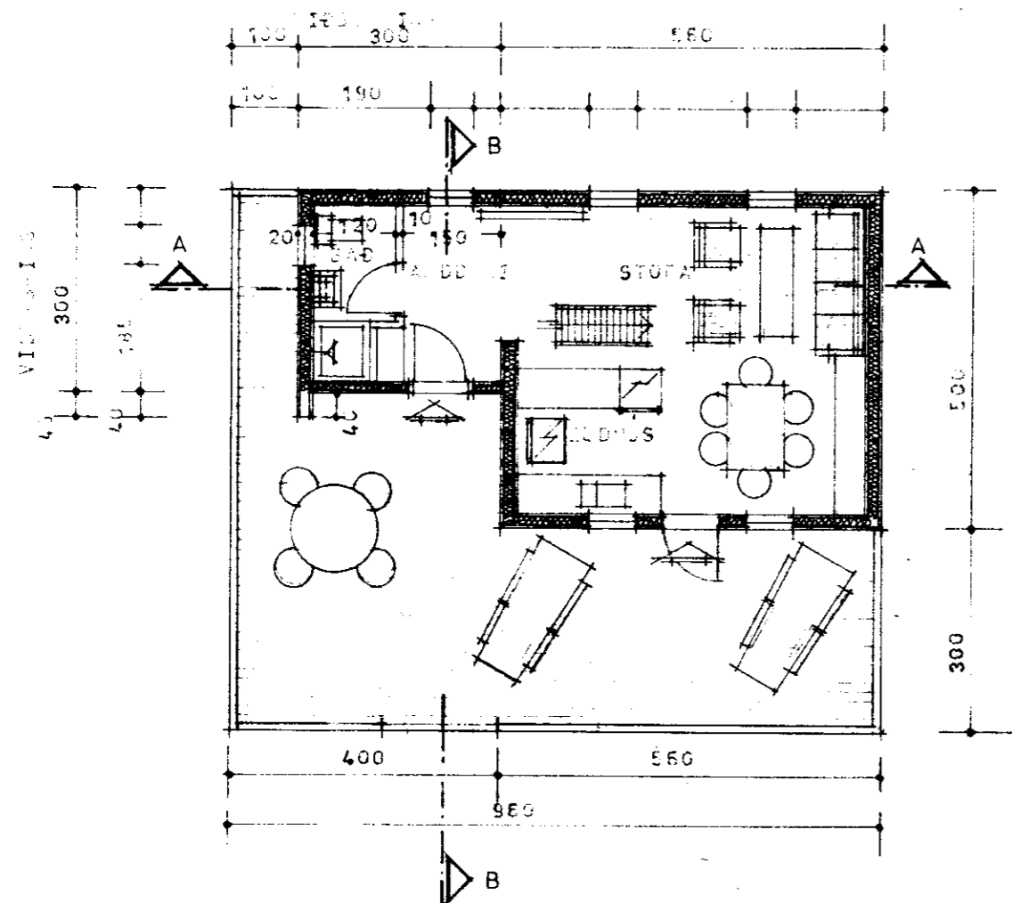
GRUNNMYND. M=1:100
