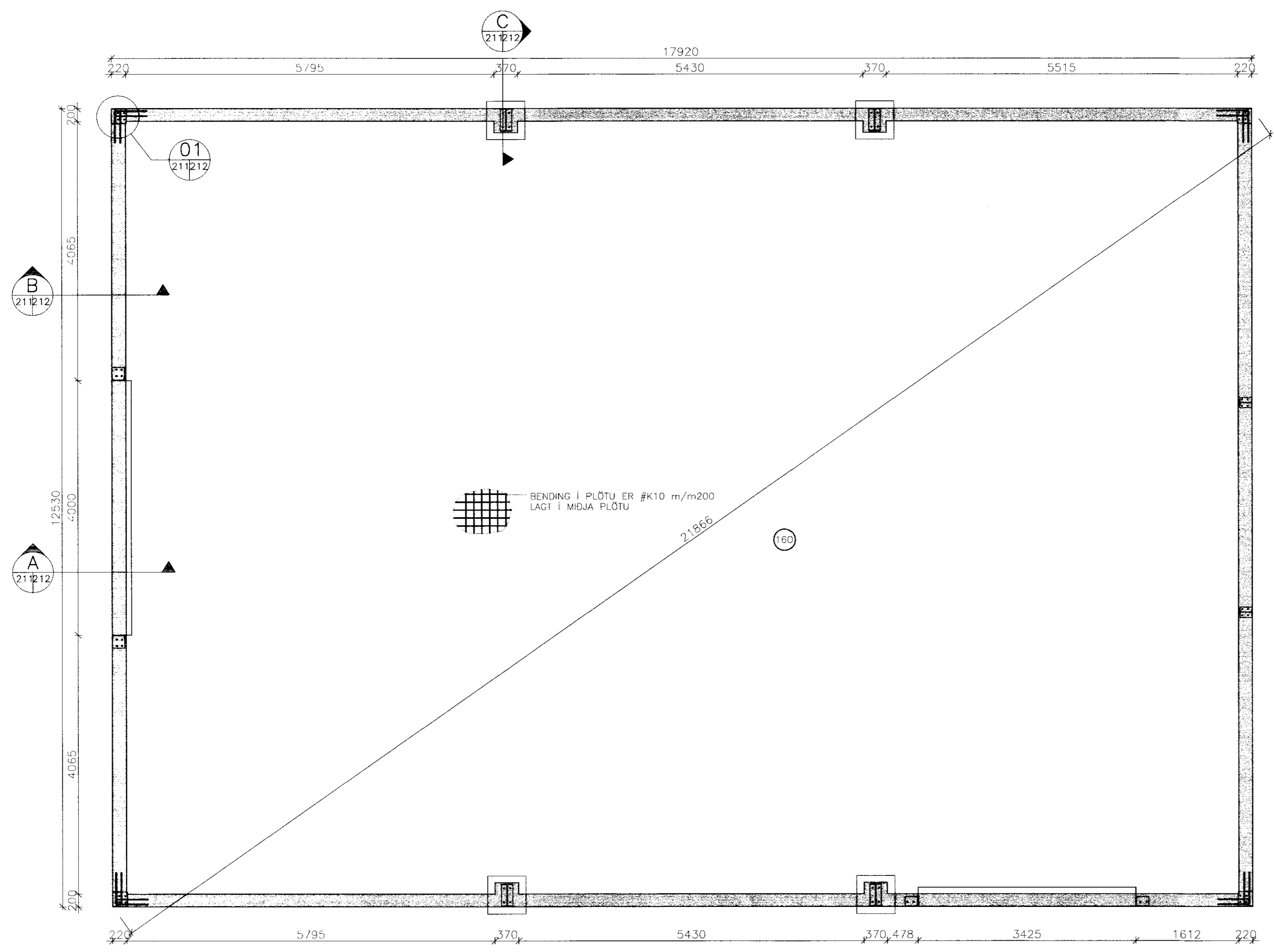
SÖKKLAR OG BOTNPLATA 1:50
