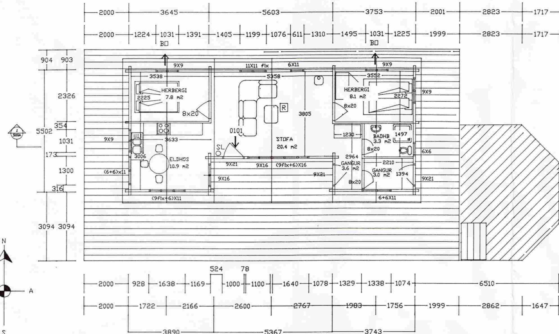
GRUNNMYND 1. HÆÐ 1:100
