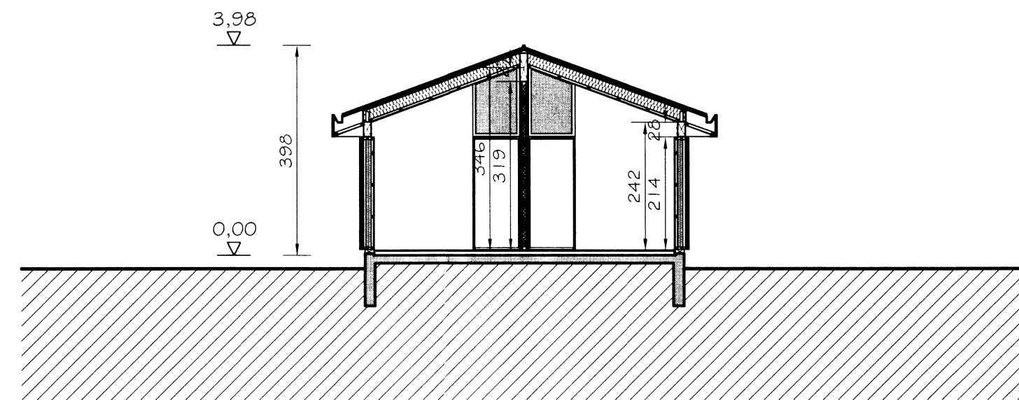
SNEIÐING C - C
