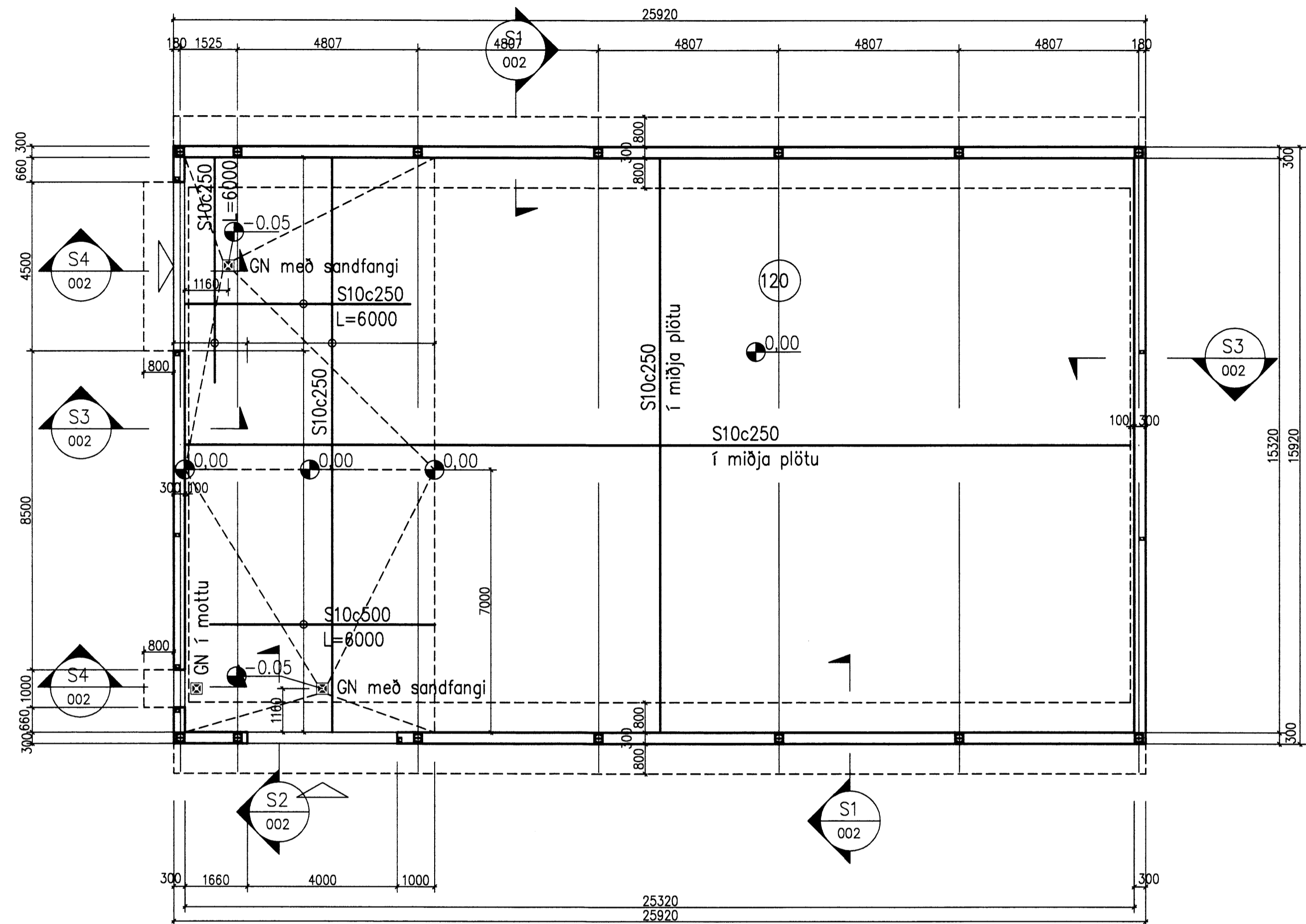
GRUNNMYND 1:100
