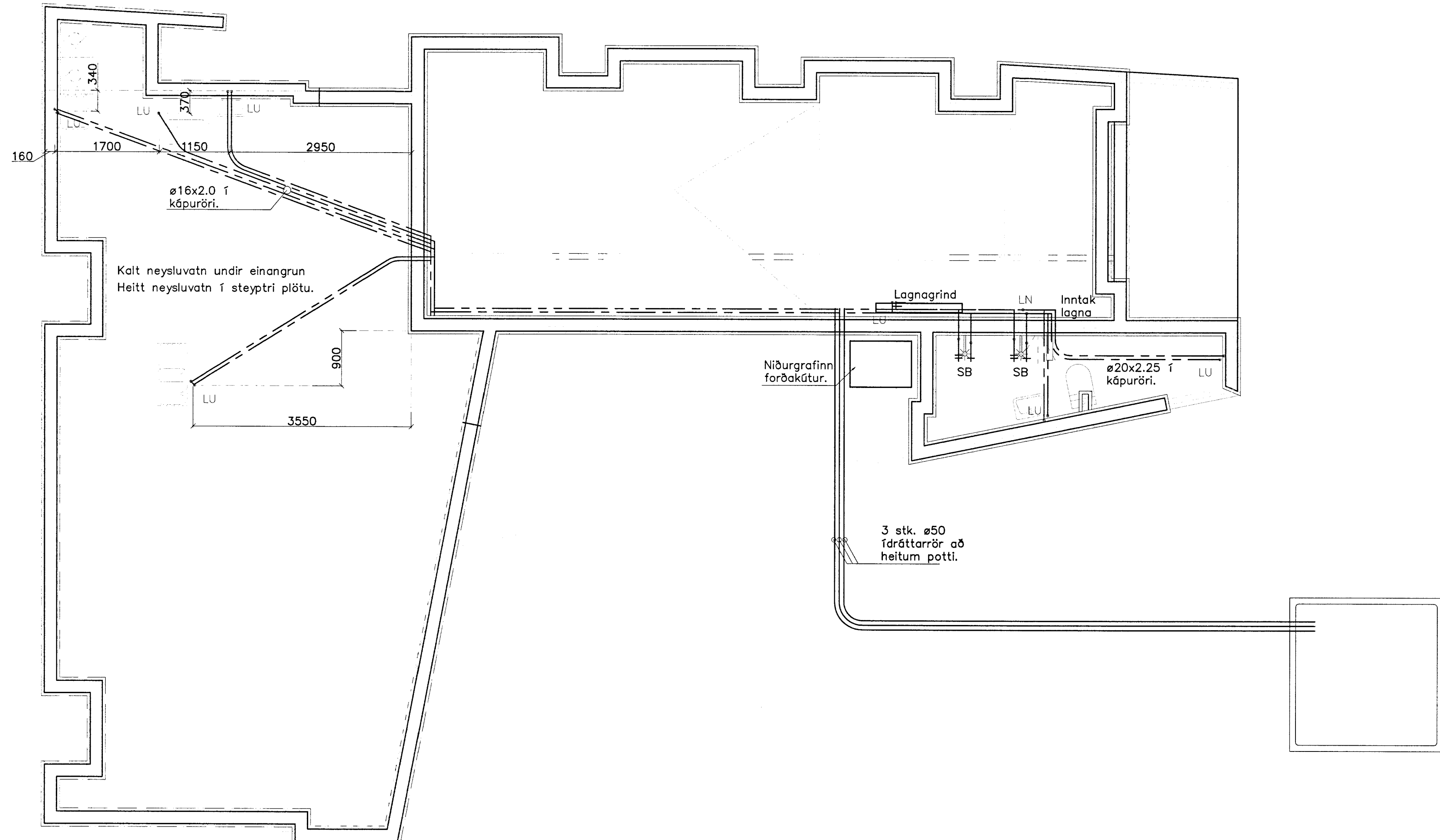
Neysluvatnslangir kjallara Mkv. 1:50
