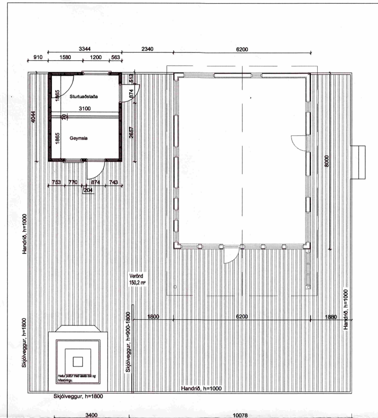
Grunnmynd 1:100
