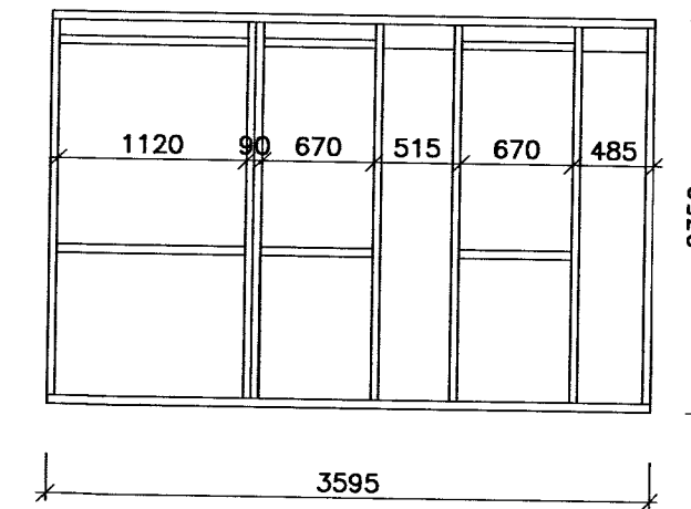
VEGGUR (5) 1:50
