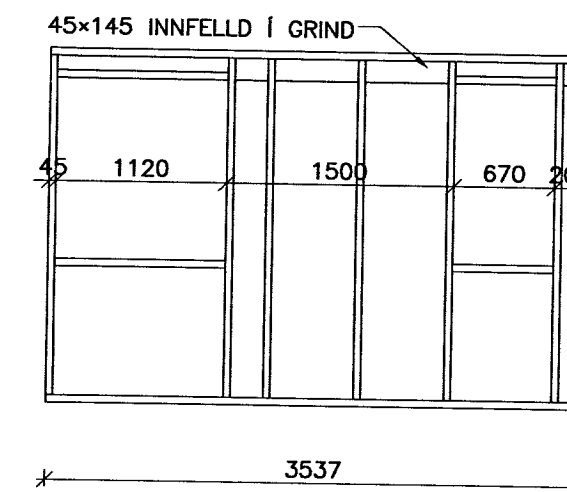
VEGGUR (2) 1:50
