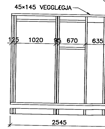
VEGGUR (6) 1:50
