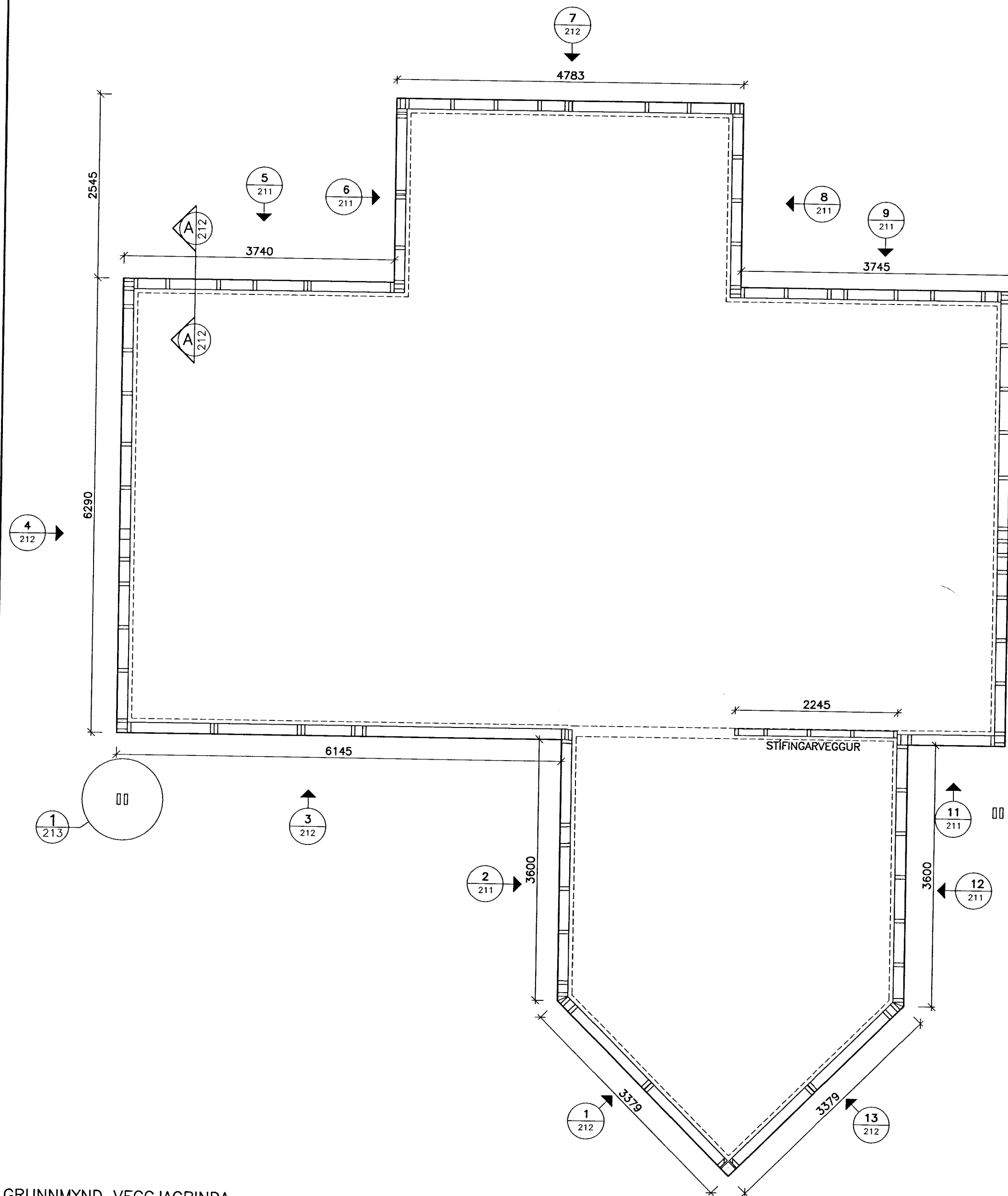
GRUNNMYND VEGGJAGRINDA Mkv 1:50
