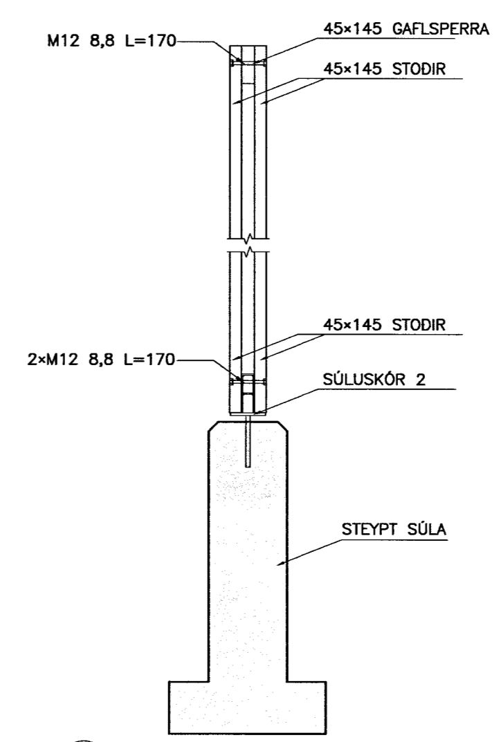
DEILI 1 1:20
