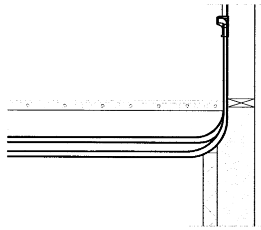
STADSETNING STÚTA VID ÚTVEGG Mkv. 1:20
