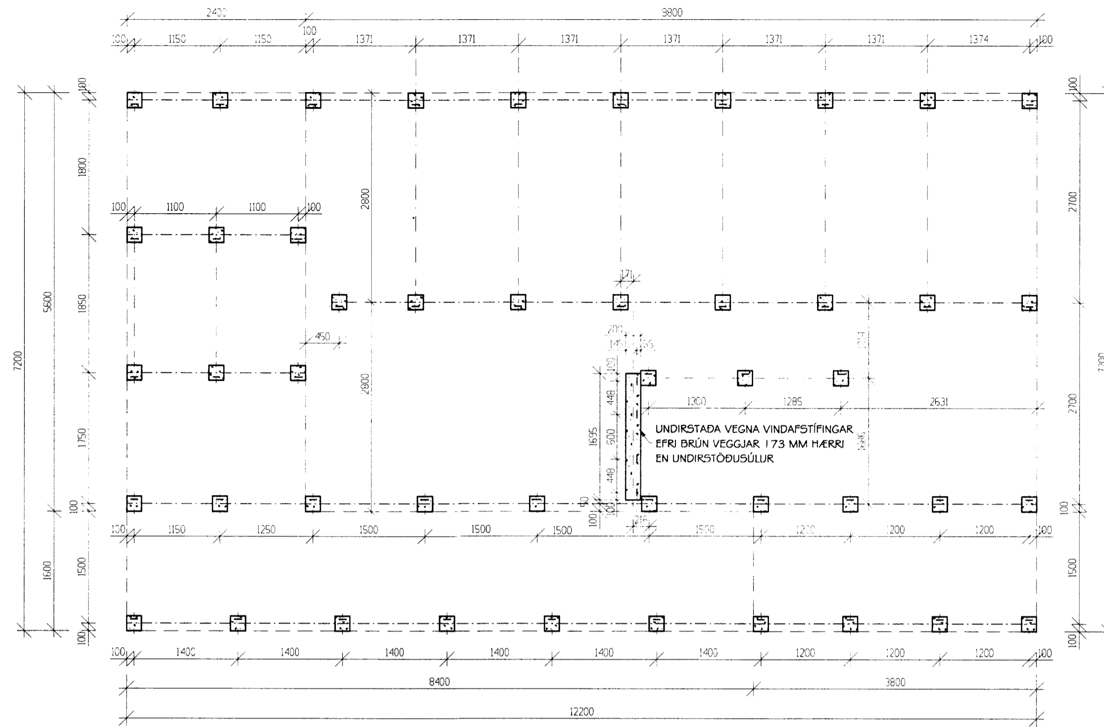
UNDIRSTÖÐUR - GRUNNMYND MKV. 1:50
