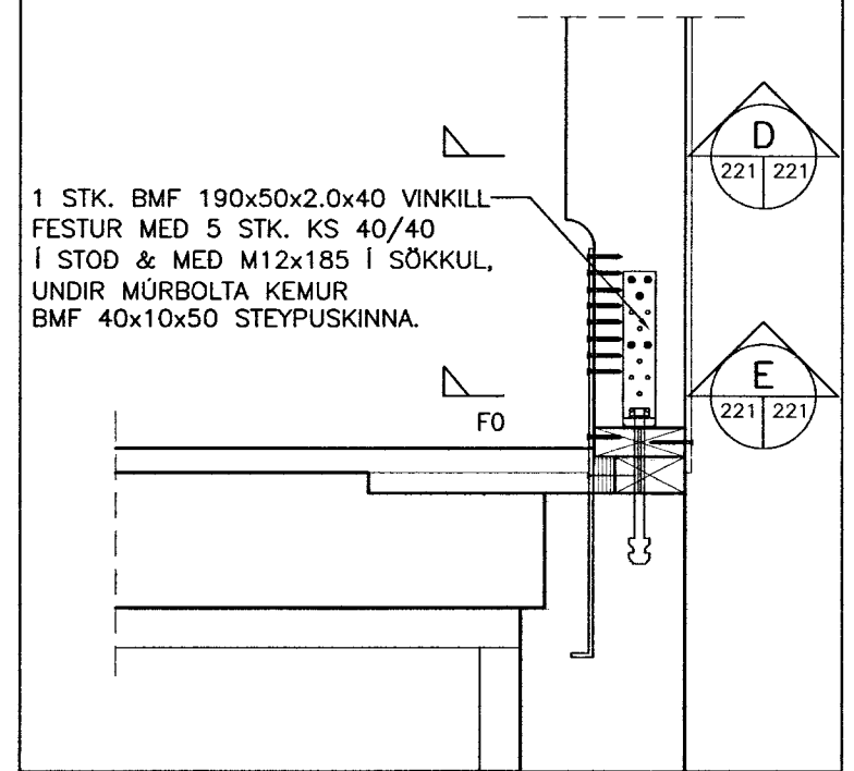
SNID E 1:10
