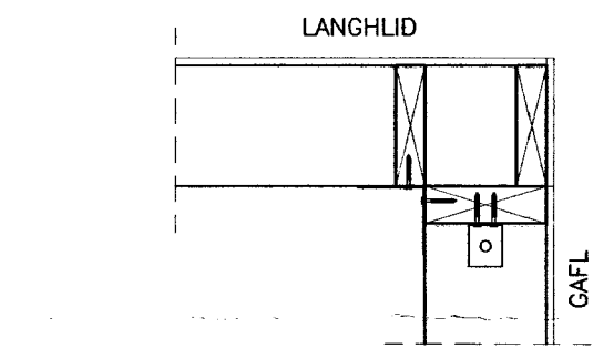
SNID E 1:10
