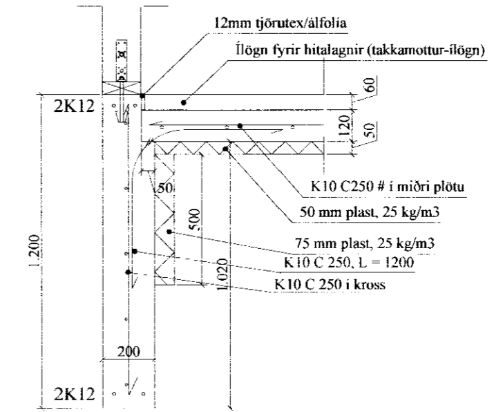
A SNID 161 1:20
