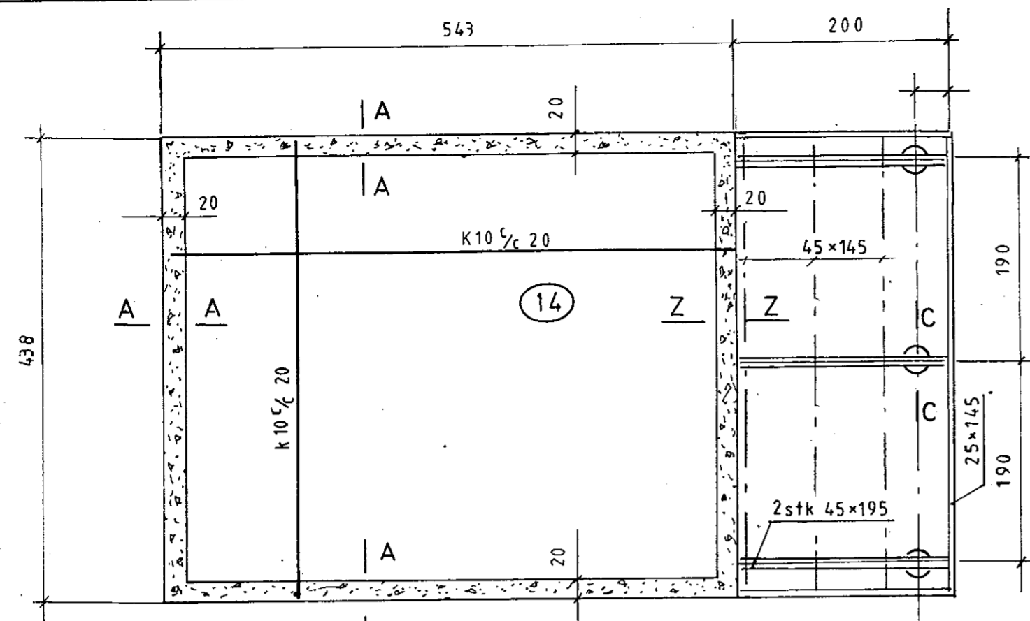
Plan sökkuls 1:50
