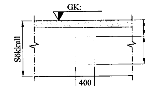
Skýringamynd af inntaksgati GK:
