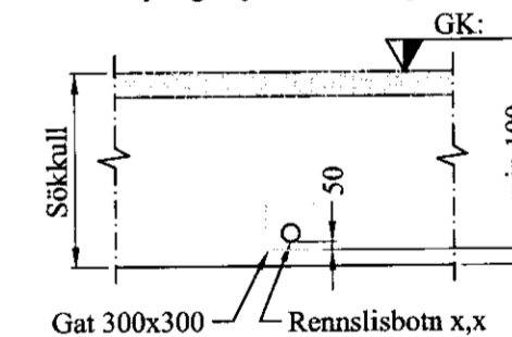
Skýringamynd af sökkulgötum GK:
