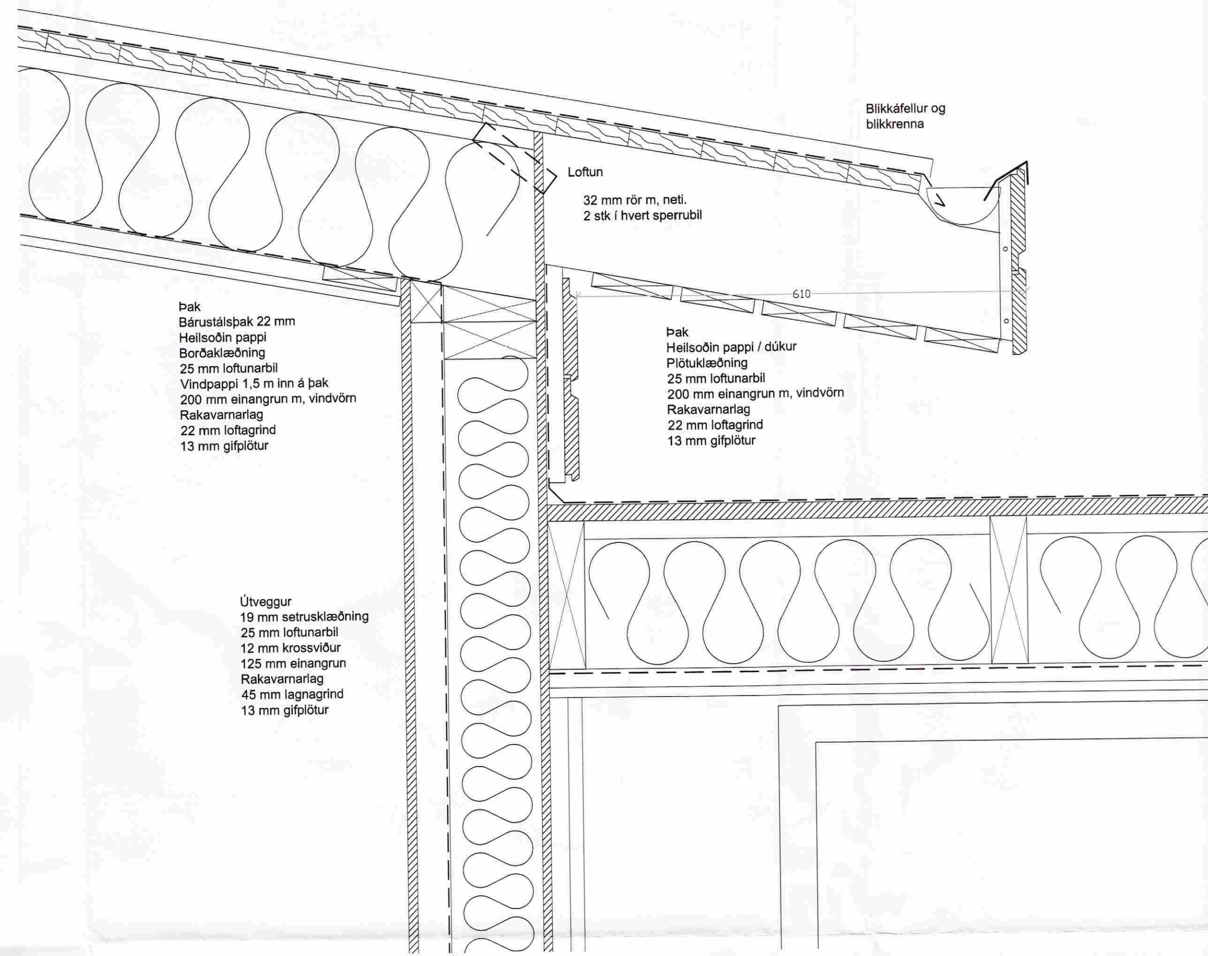
D 3 Lóðrétt sneiðing í Þakskegg mkv 1:5
