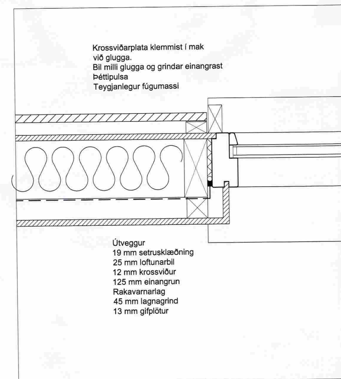
D 4 Lárétt sneiðing í Útvegg mkv 1:5
