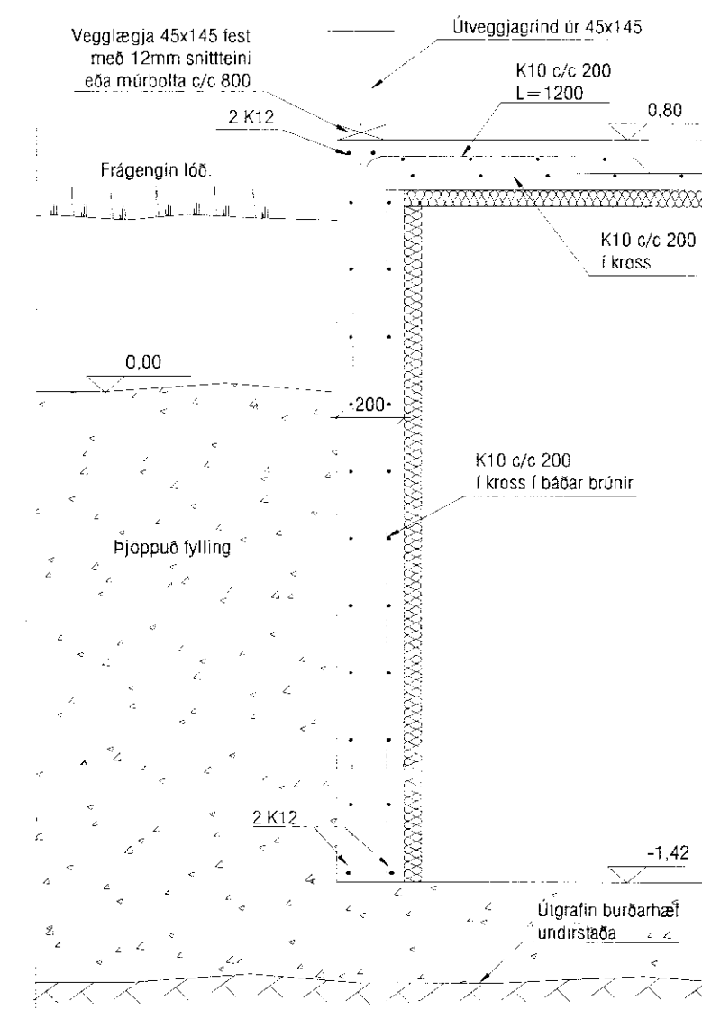
SKURÐUR A - A Í SÖKKULÚTVEGG Mv. 1:20
