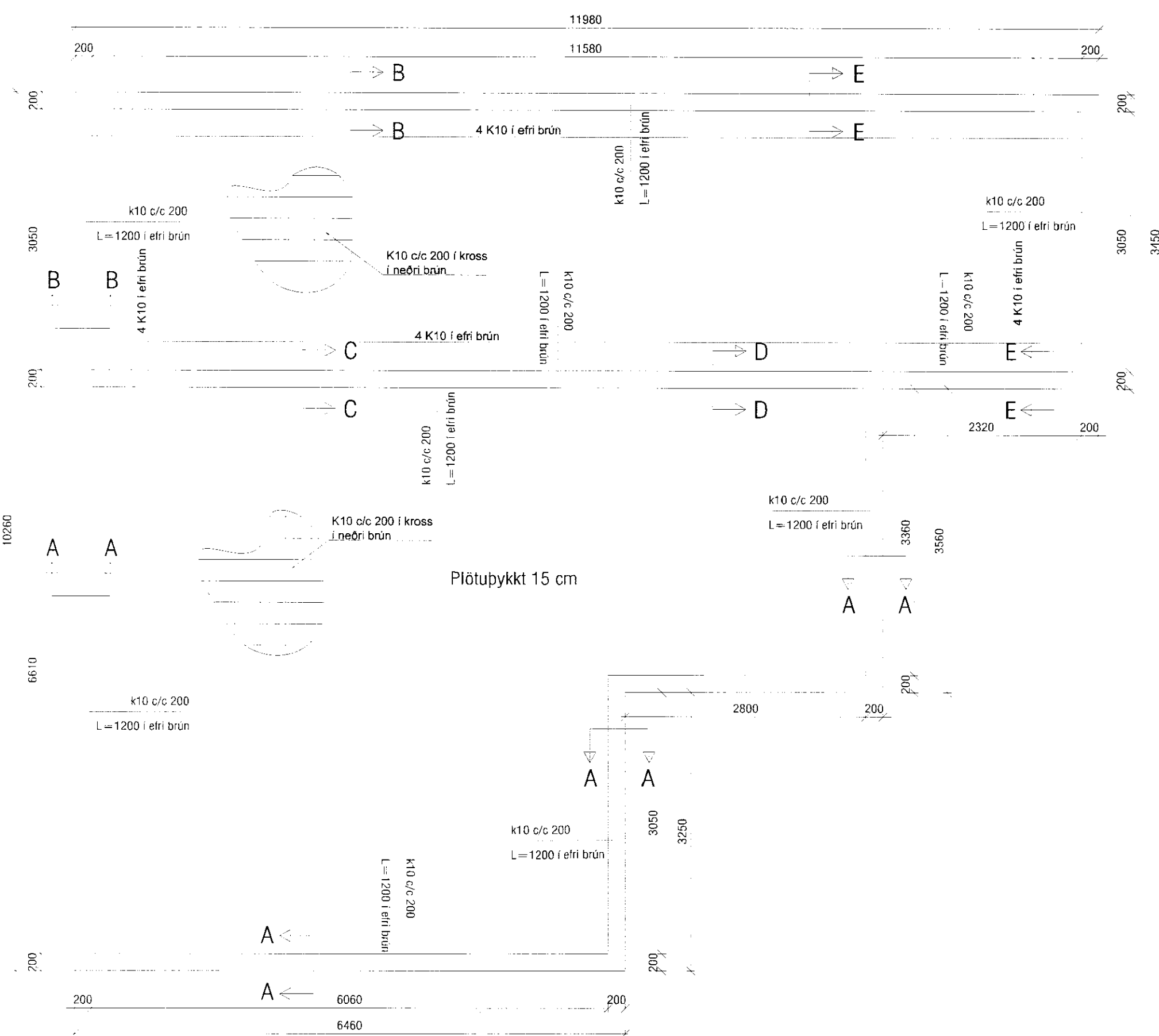
SÖKKULGRUNNMYND Mv. 1:50
