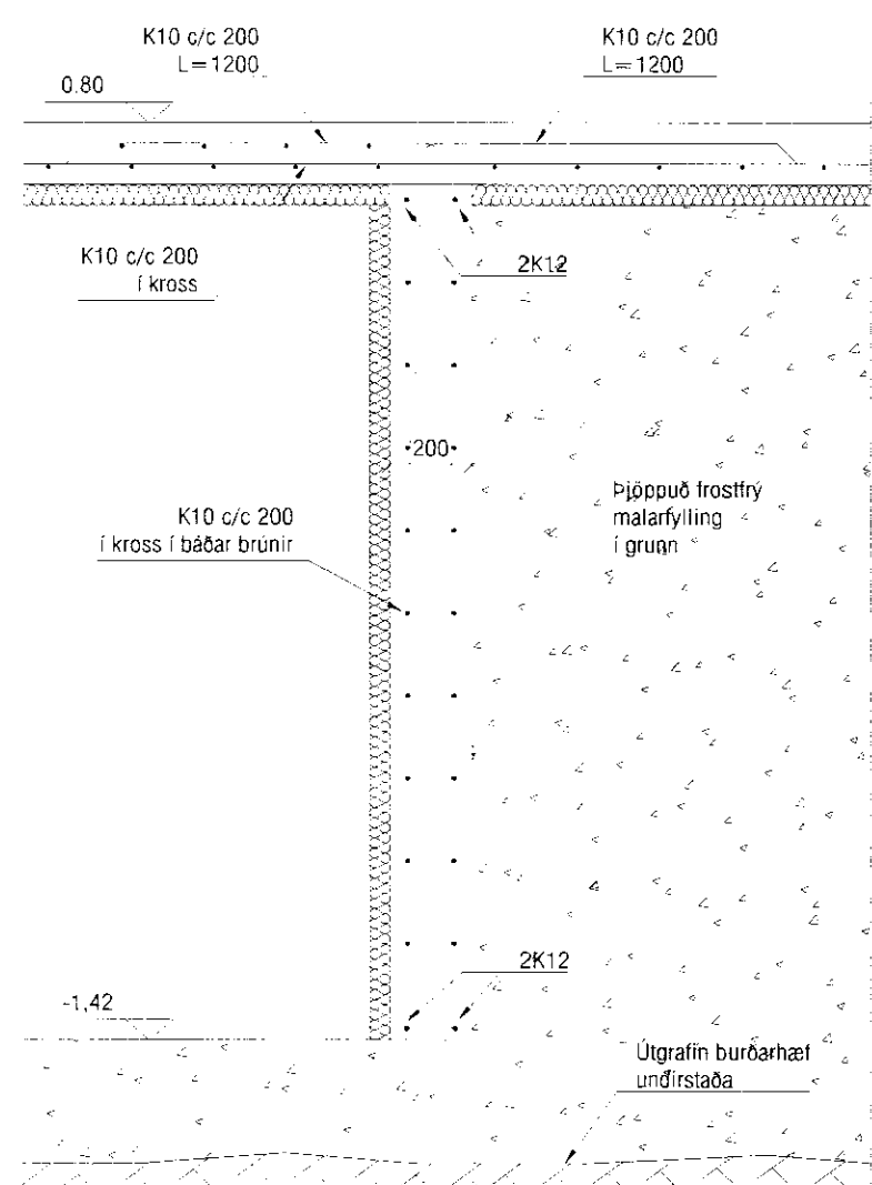
SKURÐUR C - C Í SÖKKULVEGG Mv. 1:20
