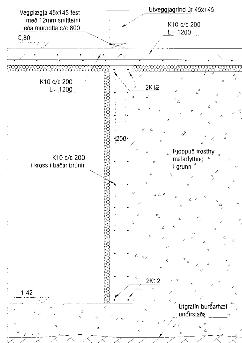
SKURÐUR D - D Í SÖKKULVEGG Mv. 1:20
