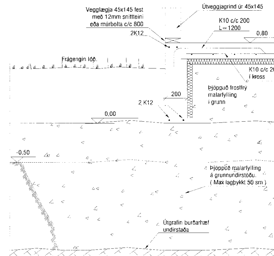
SKURÐUR A - A Í SÖKKULÚTVEGG Mv. 1:20
