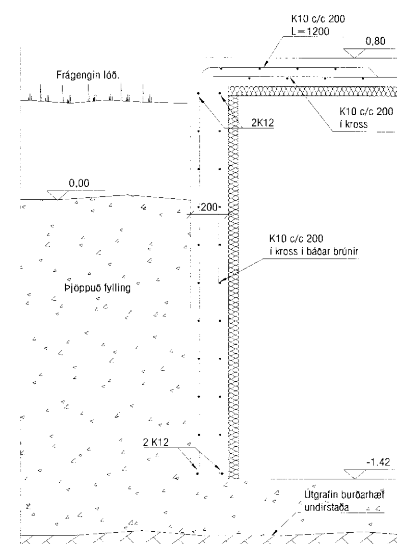
SKURÐUR E - E Í SÖKKULVEGG Mv. 1:20
