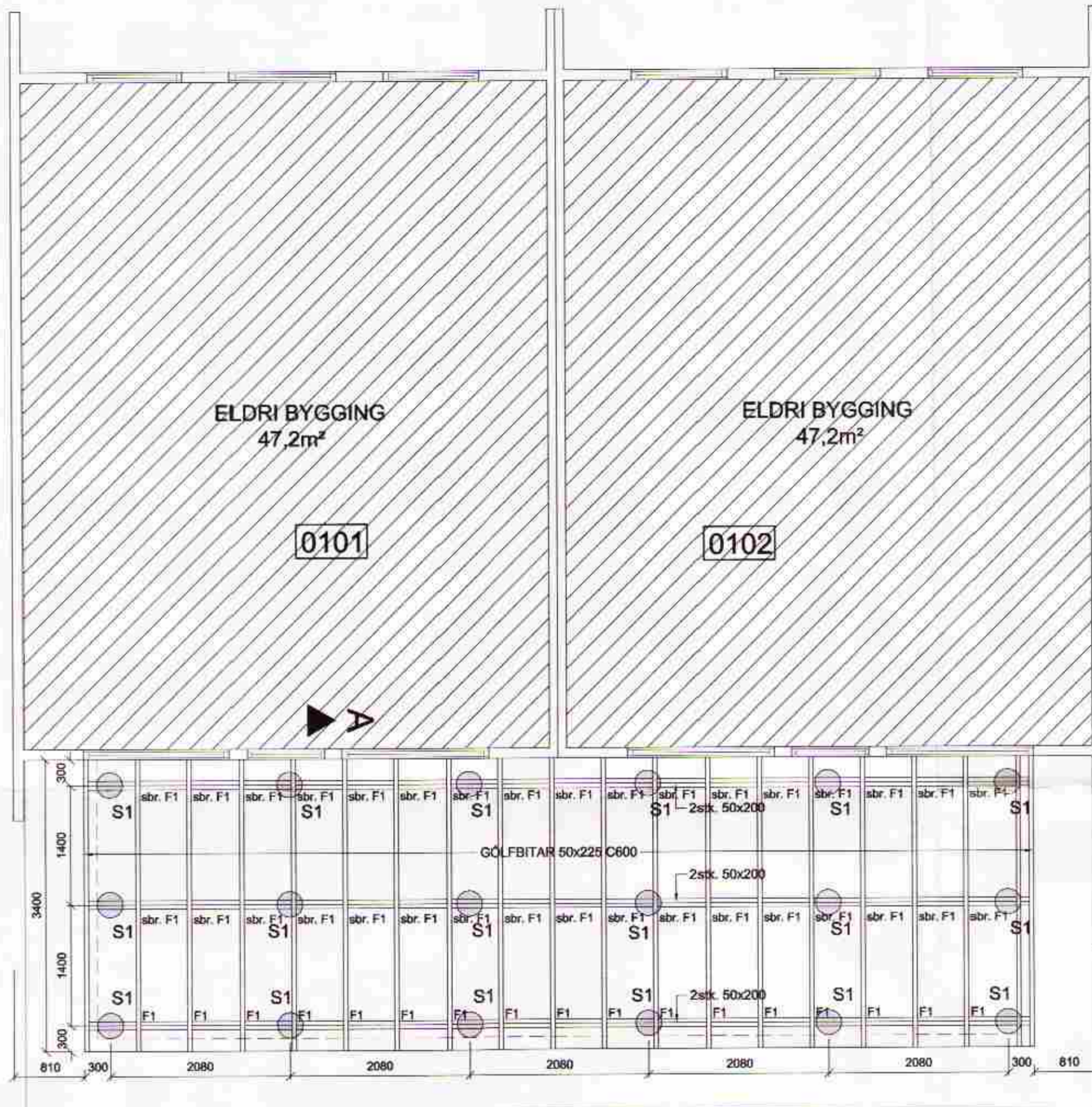
GRUNNMYND GÓLFBITA 1:50
