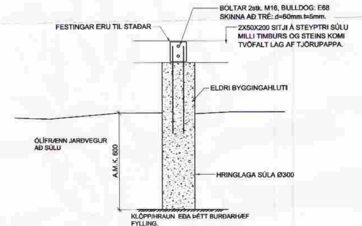
SÜLUUNDIRSTAÐA, S1: 1:20
