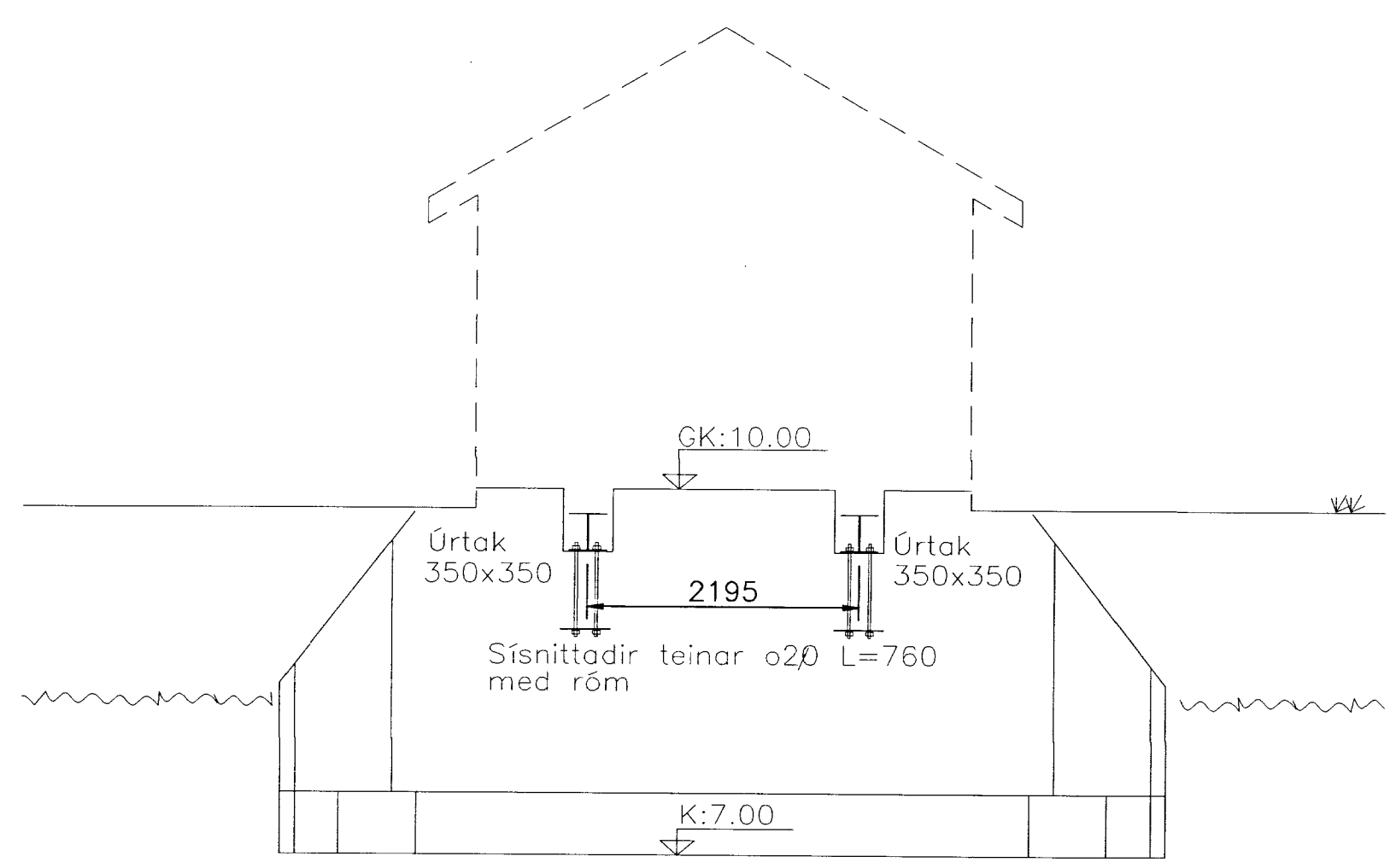
Ásýnd að utanverðu Mkv. 1:50
