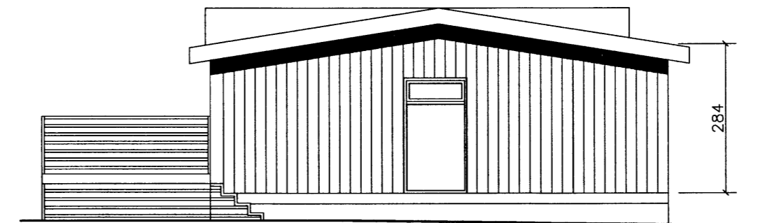
útlit austur
