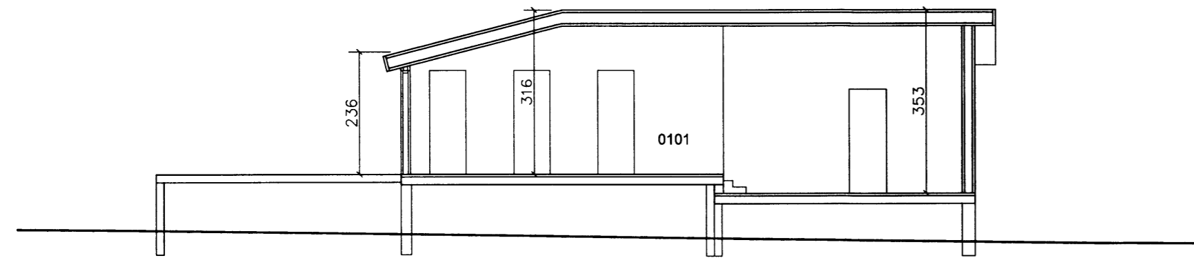
skurður A-A
