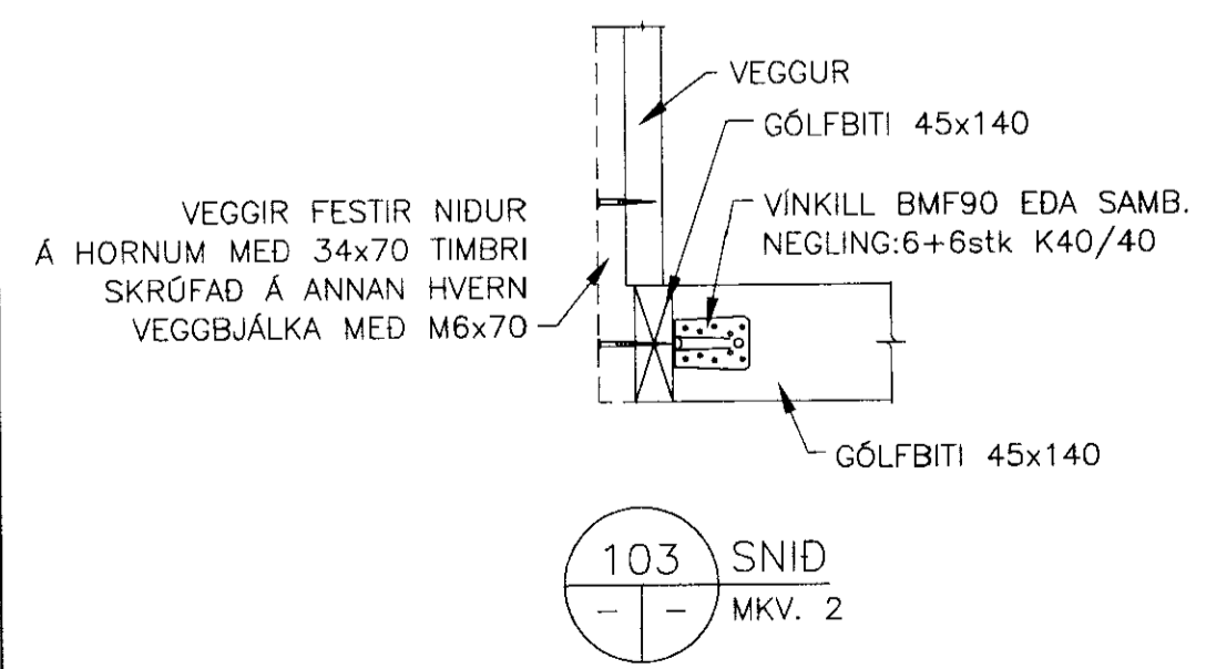
GRUNNMYND-GÓLF MKV. 1
