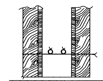
Snið í sökkulvegg Sýnd eru 2 neöstu steypu- styrktarjárni í steypunóti ofan á neöstu nótavirnum.
