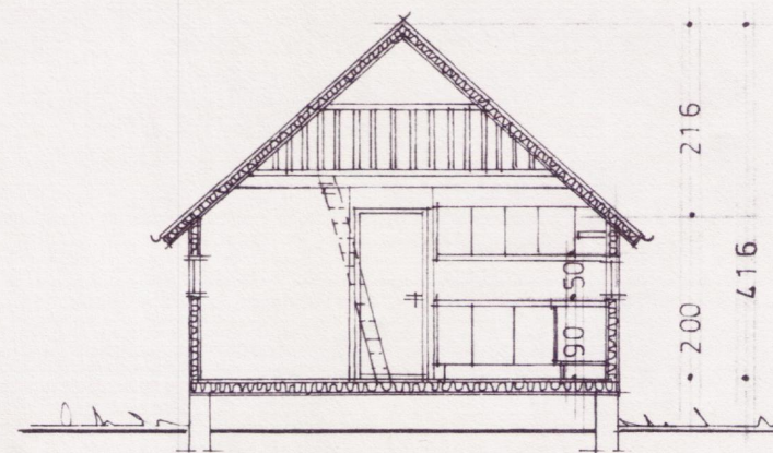
SNIÐ
