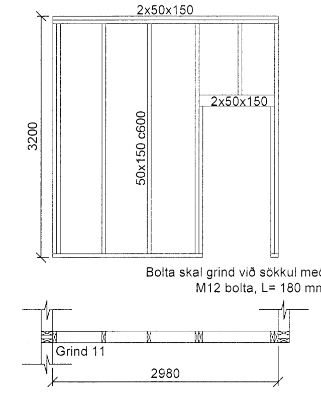
Grind nr. 11 - Séð utan frá Mkv. 1:50
