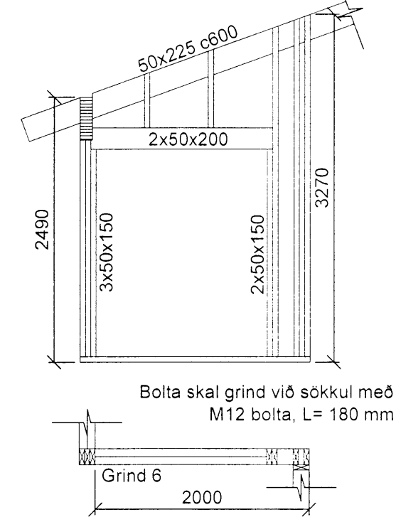
Grind nr. 6 - Séð utan frá Mkv. 1:50
