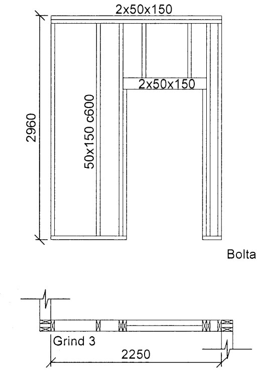
Grind nr. 3 - Séð utan frá Mkv. 1:50
