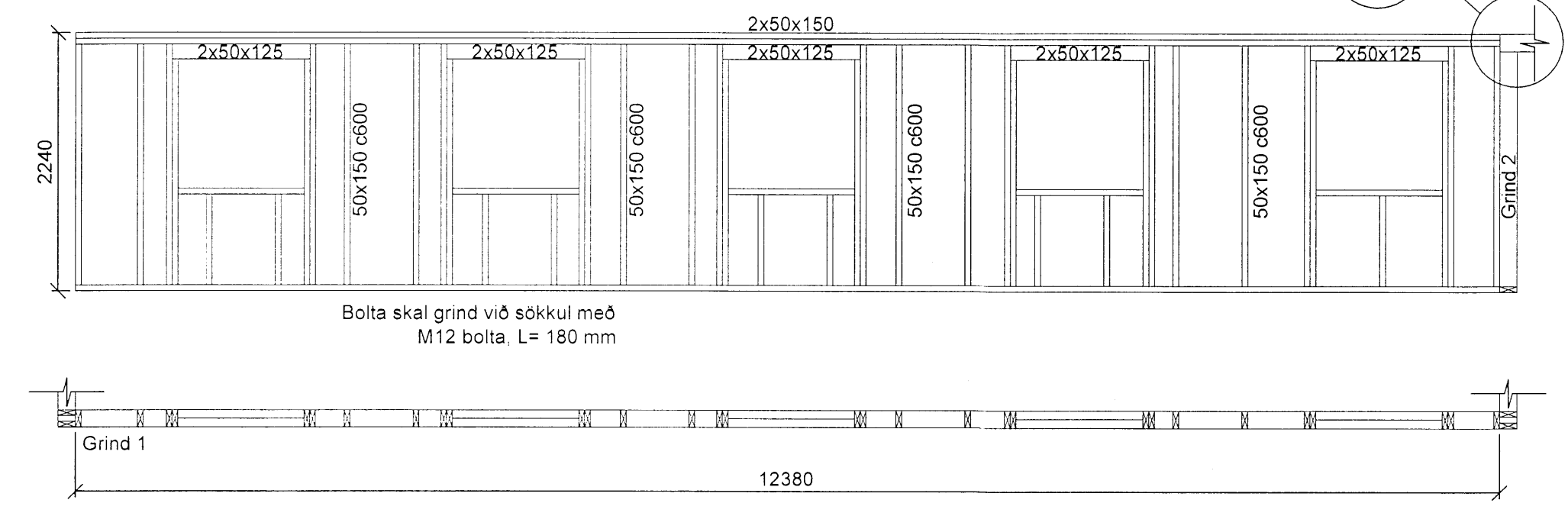
Grind nr. 1 - Séð utan frá Mkv. 1:50
