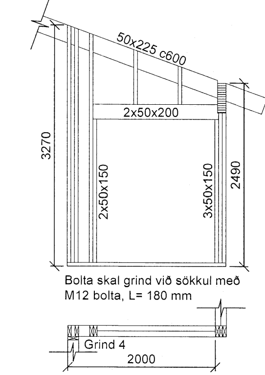
Grind nr. 4 - Séð utan frá Mkv. 1:50
