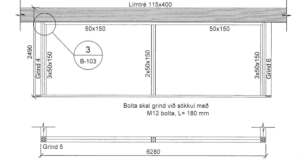
Grind nr. 5 - Séð utan frá Mkv. 1:50
