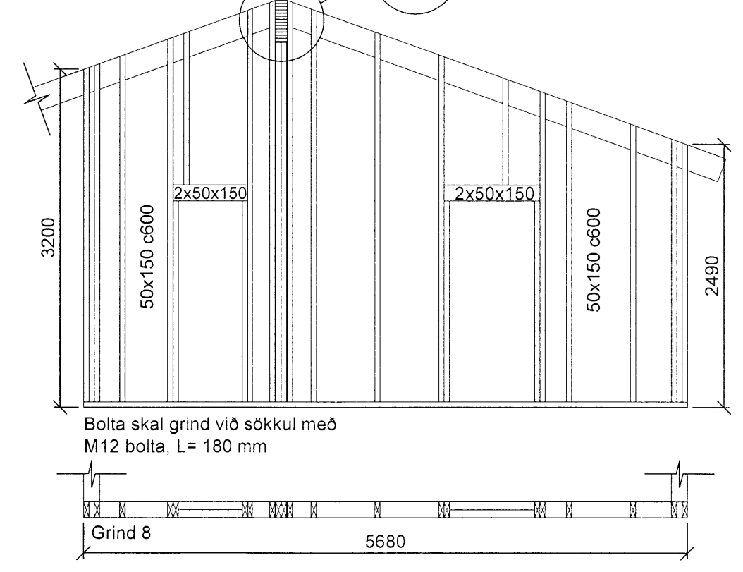
Grind nr. 8 - Séð utan frá Mkv. 1:50
