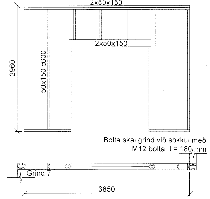
Grind nr. 7 - Séð utan frá Mkv. 1:50
