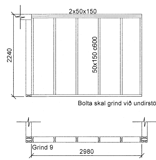
Grind nr. 9 - Séð utan frá Mkv. 1:50
