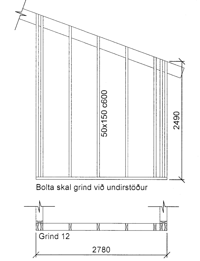
Grind nr. 12 - Séð utan frá Mkv. 1:50
