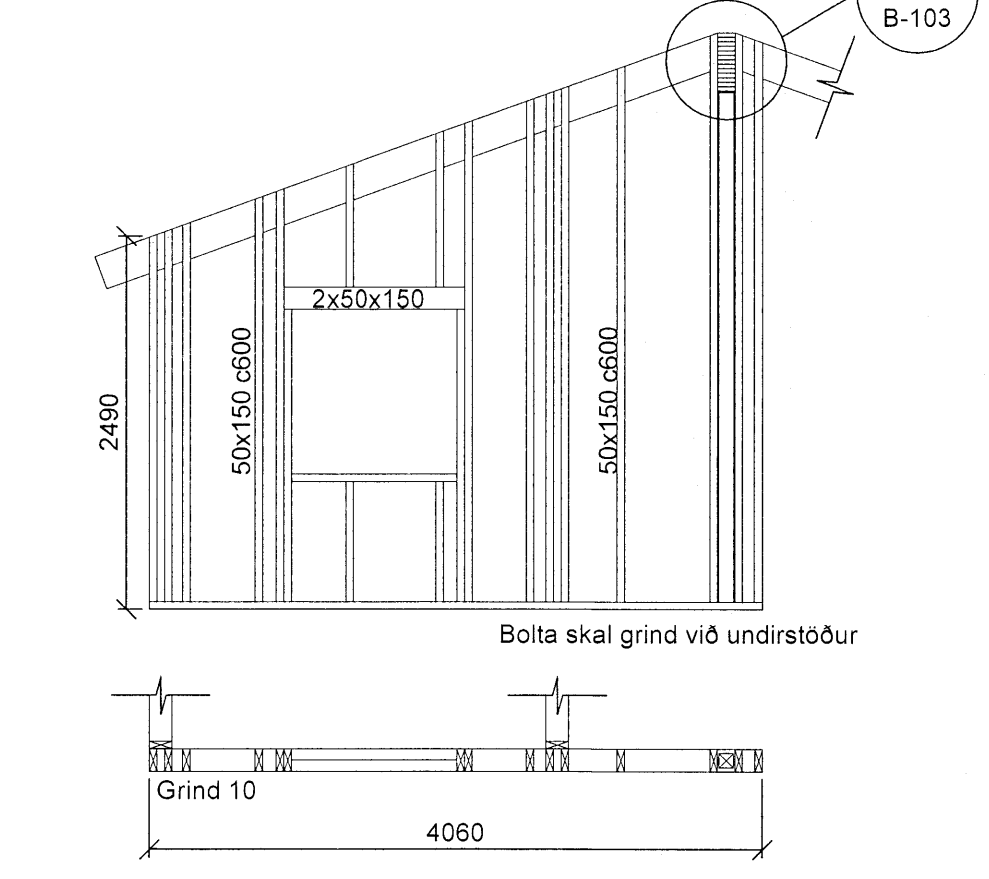
Grind nr. 10 - Séð utan frá Mkv. 1:50
